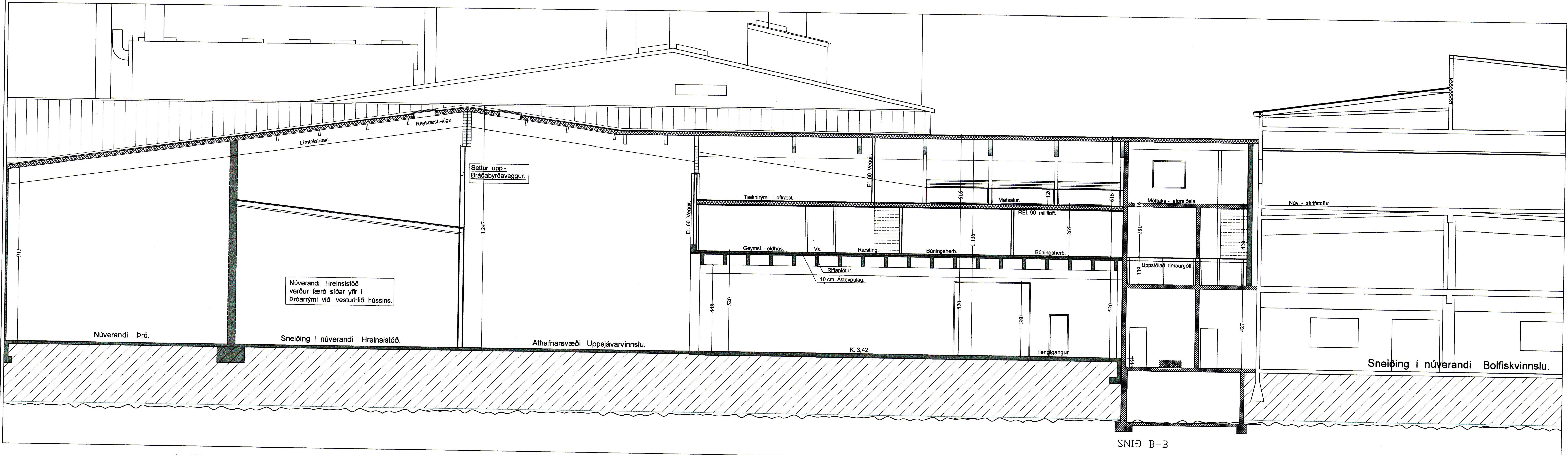
Sneiðing í viðbyggingu yfir Hfnargötu. B-B 1:100
