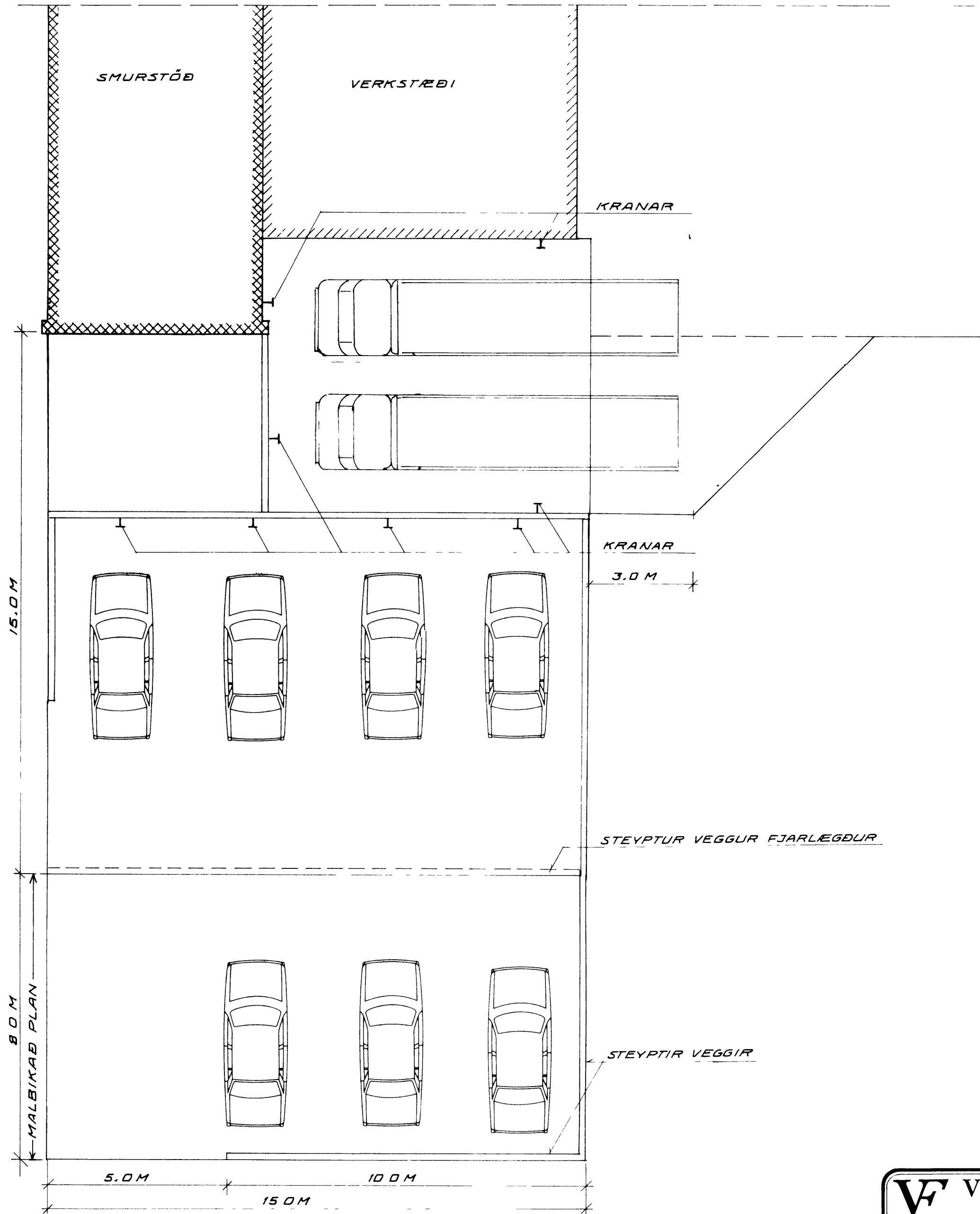
GRUNNMYND M 1:100
