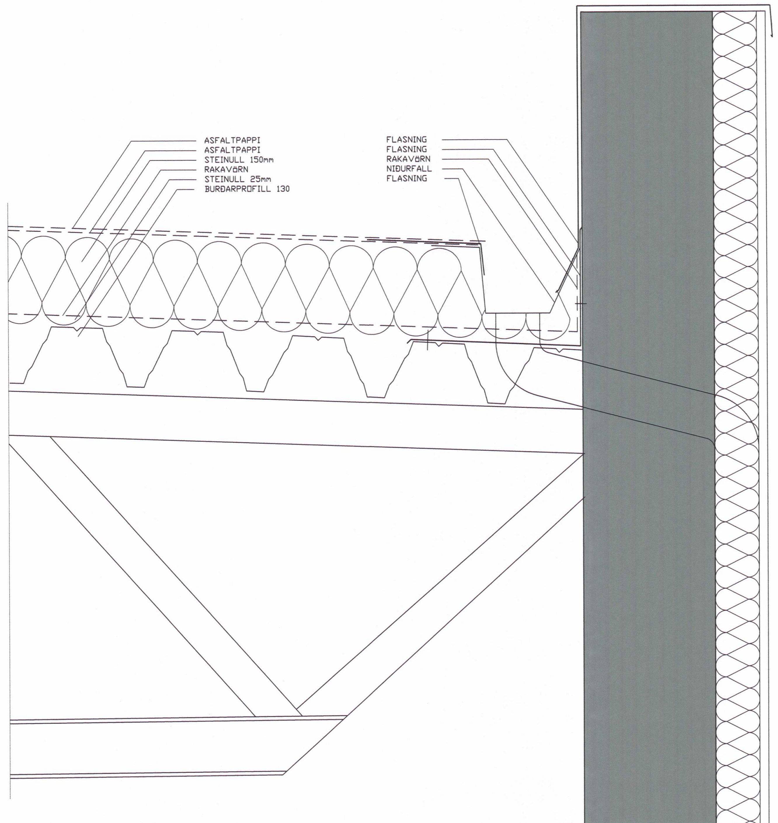
FRÁGANGUR ÞAKS VIÐ NIÐURFÖLL
