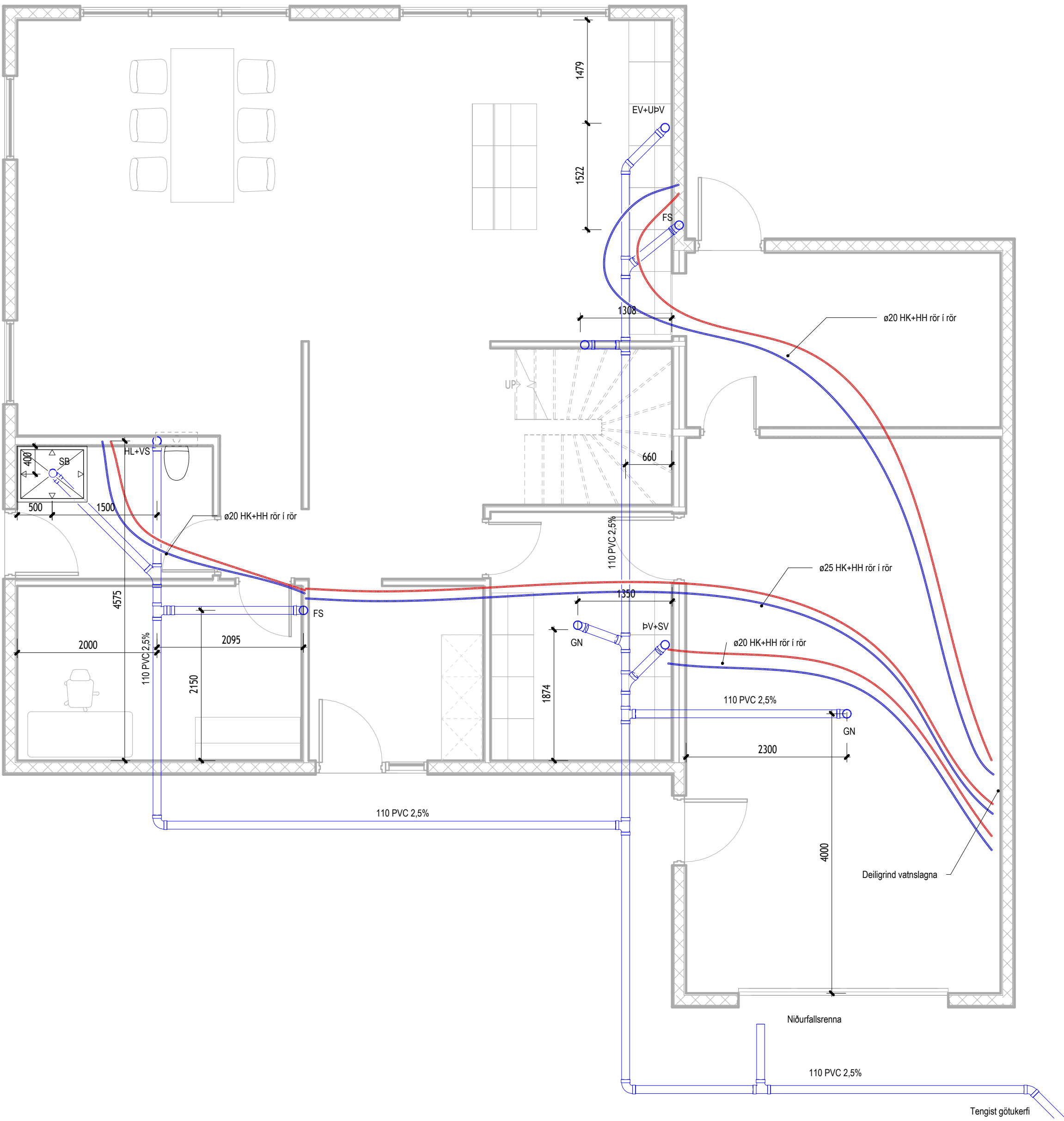
Grunnmynd - Grunnlagirnir mkv: 1 : 50
