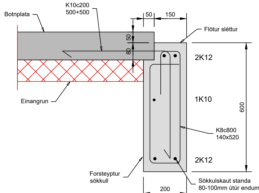
Snið 01
