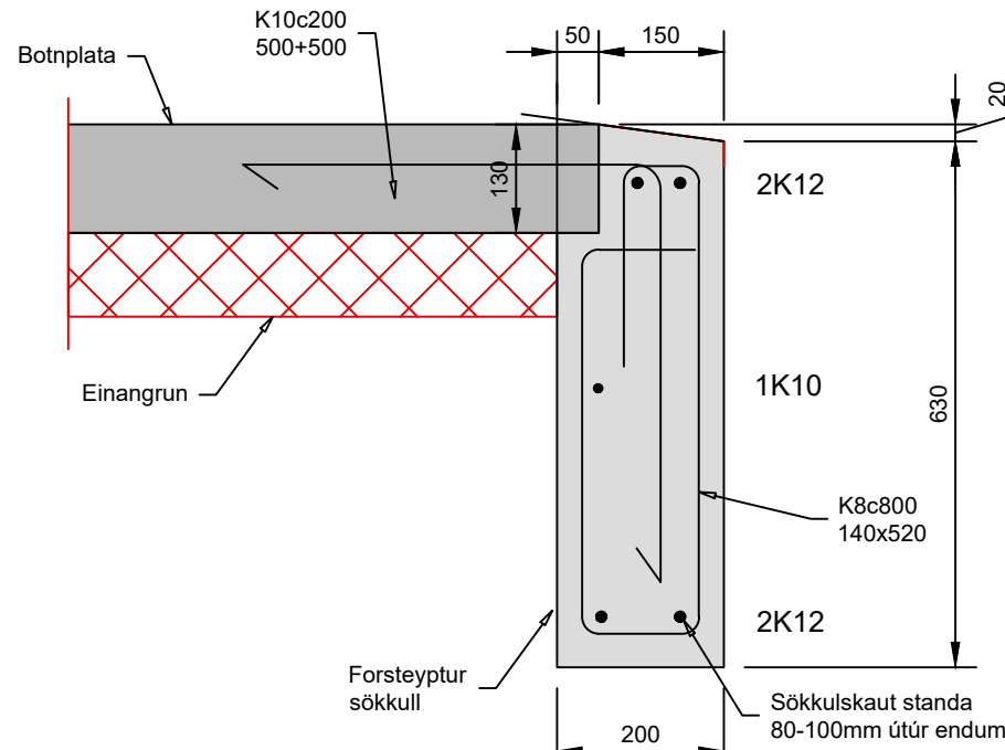
Snið 02 (bílskúrgat)
