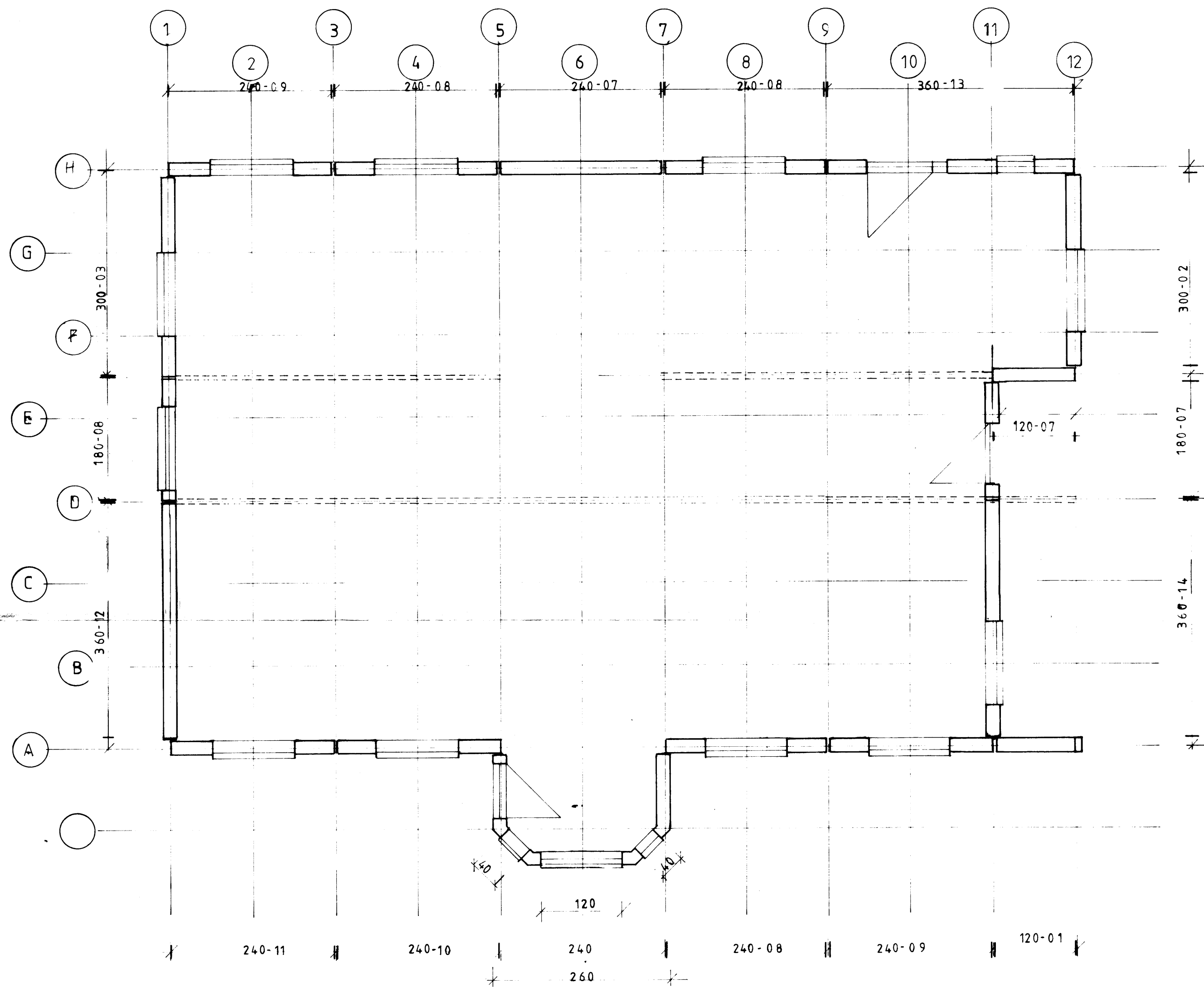
GRUNNMYND 1:50
