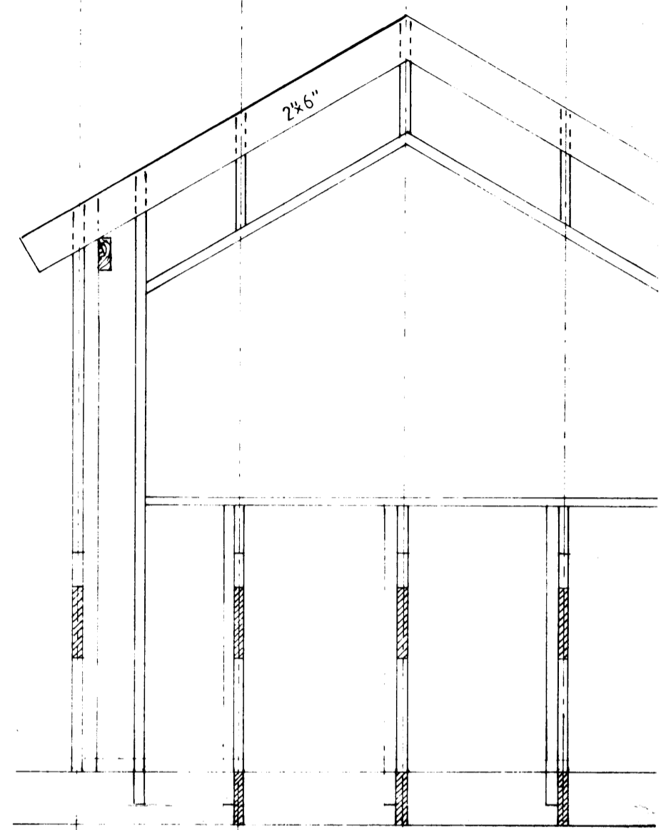
Kvistur snið B-B 120
