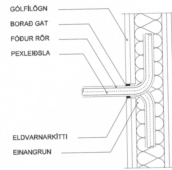
BRUNAPÉTTING Á PEXLEIÐSLU Í FÓÐURRÖRI Í GEGNUM KLÆÐNINGU
