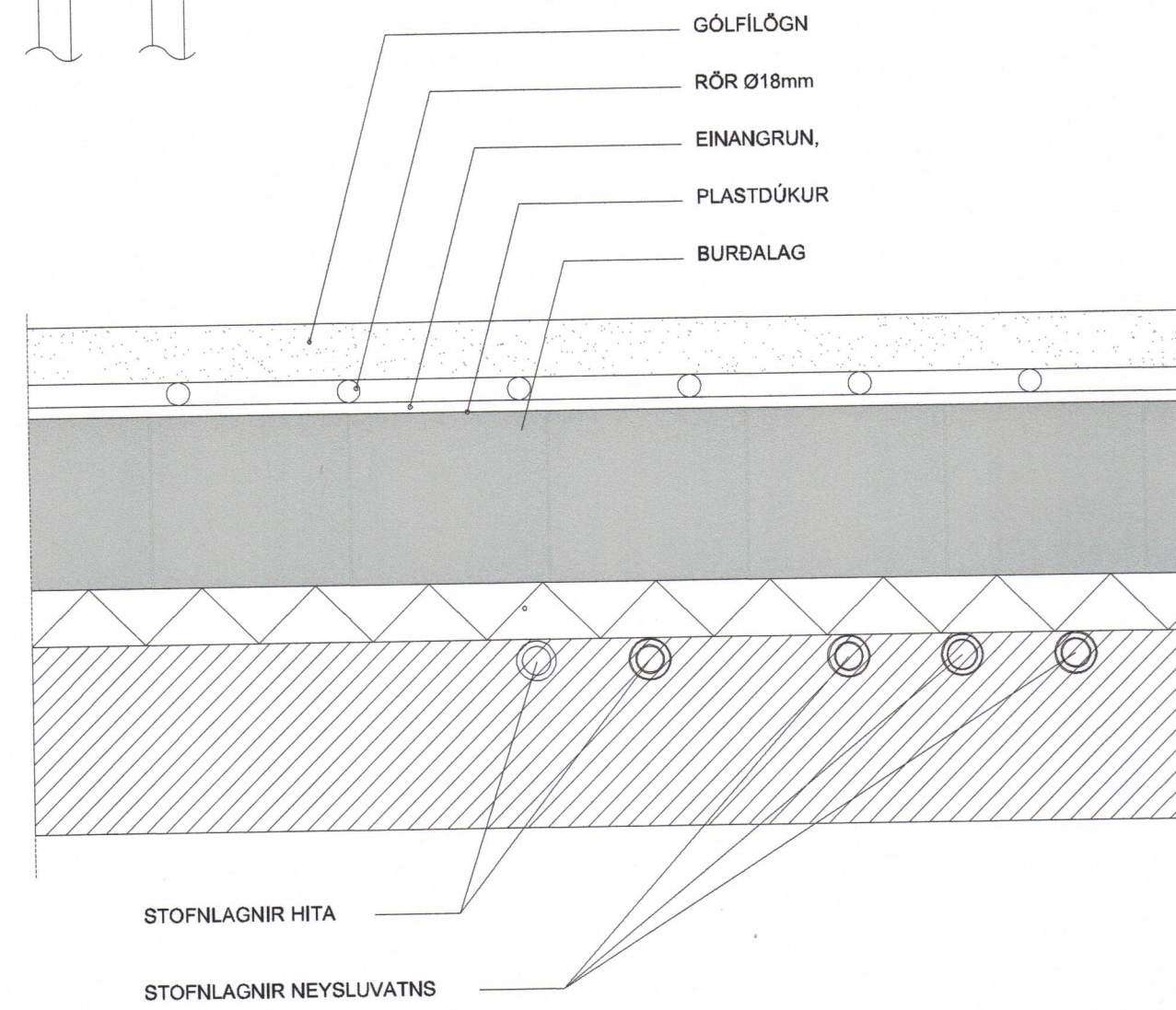
FRÁGANGUR LAGNA Í GÓLFI
