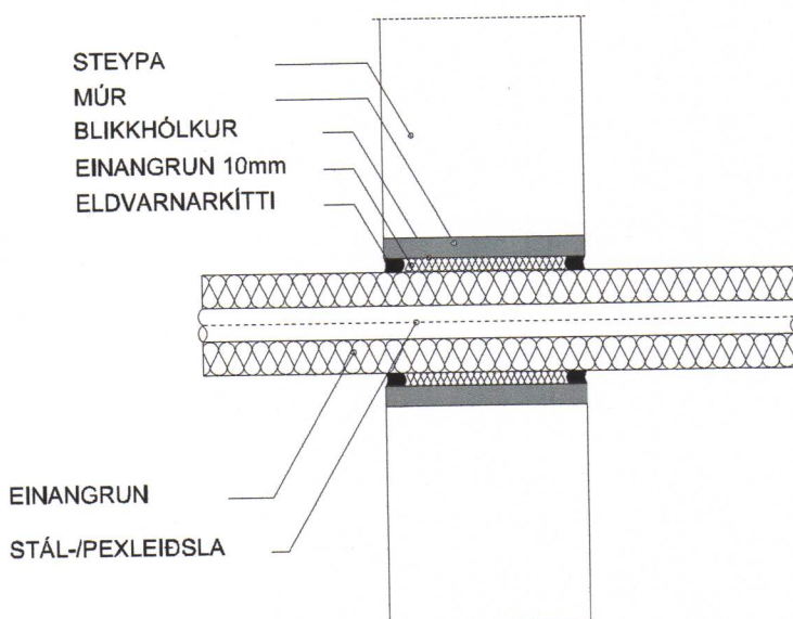
FRÁGANGUR Á STÁL-PEXLEIÐSLU GEGNUM STEYPTAN VEGG
