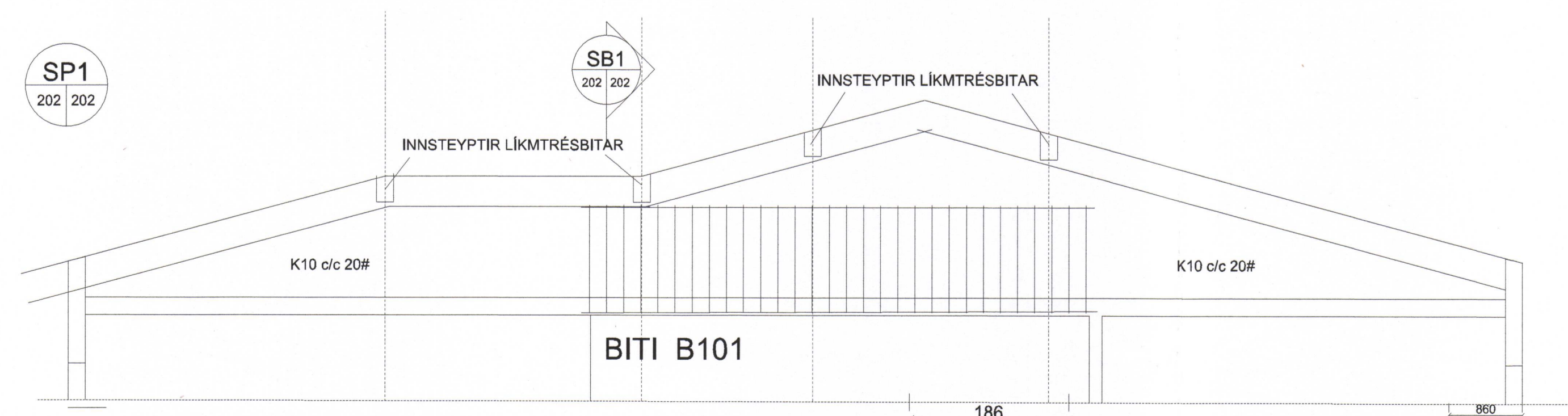
GRUNNMYND 1 HÆÐ PLATA
