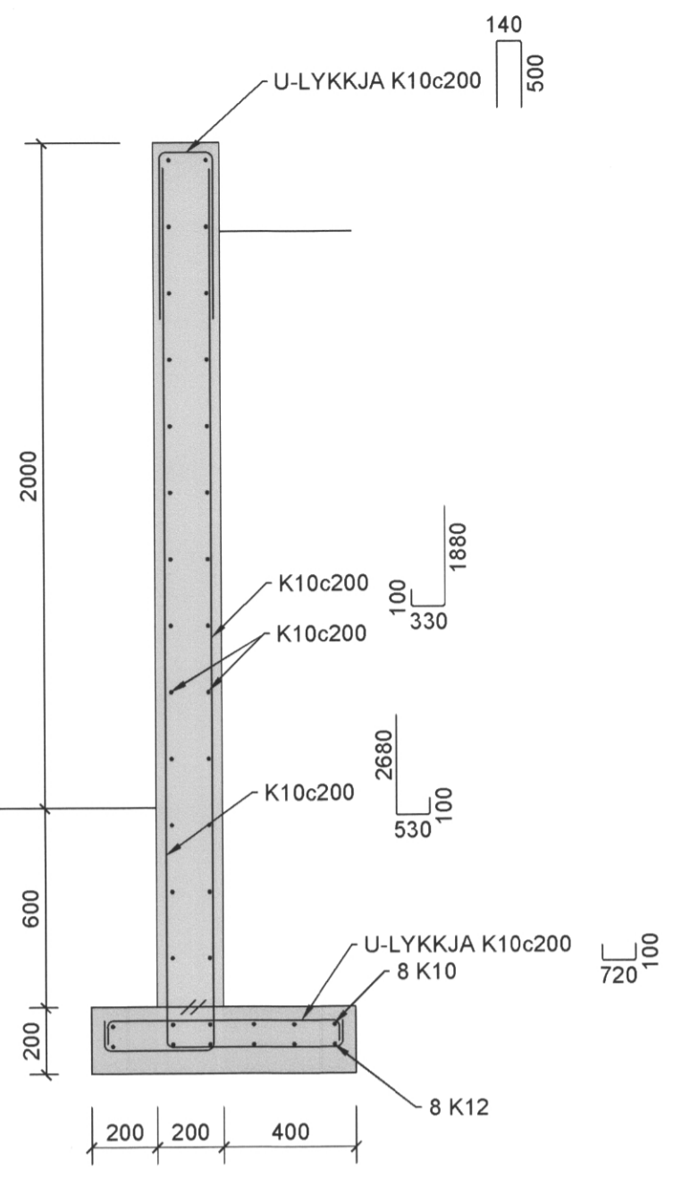
STÖÐVEGGUR Í NORÐURENDA LÓÐAR 1:20
