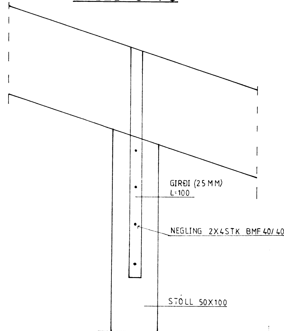
DEILI 3 1:5
