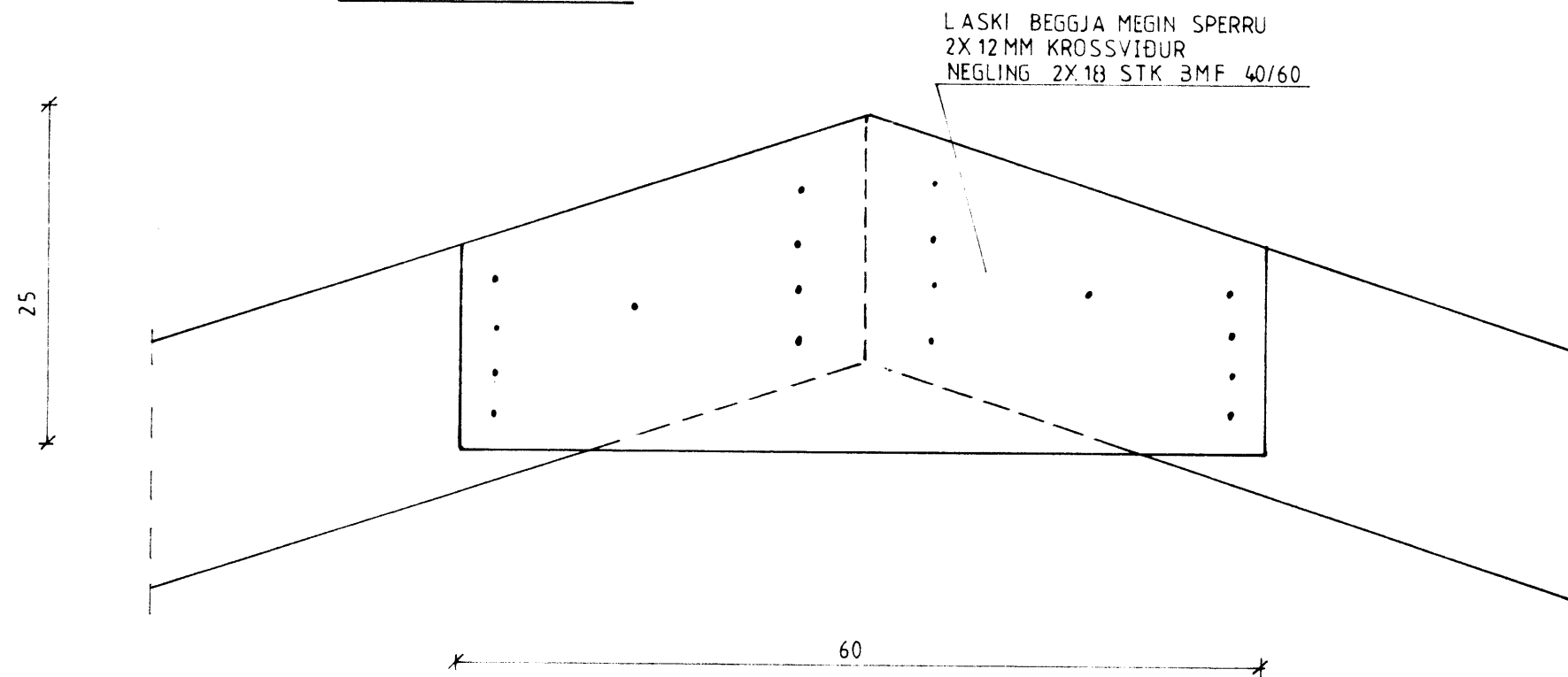
DEILI 2 1:5
