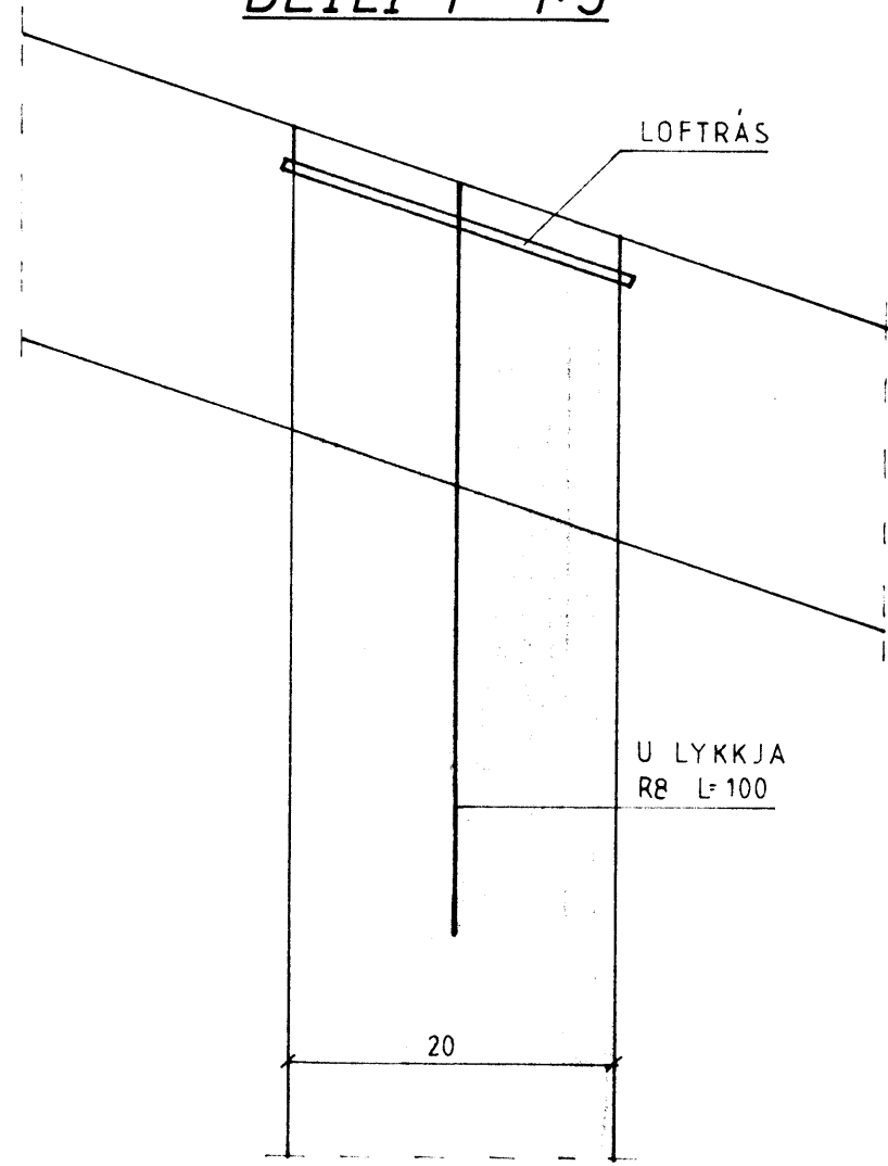
DEILI 1 1:5
