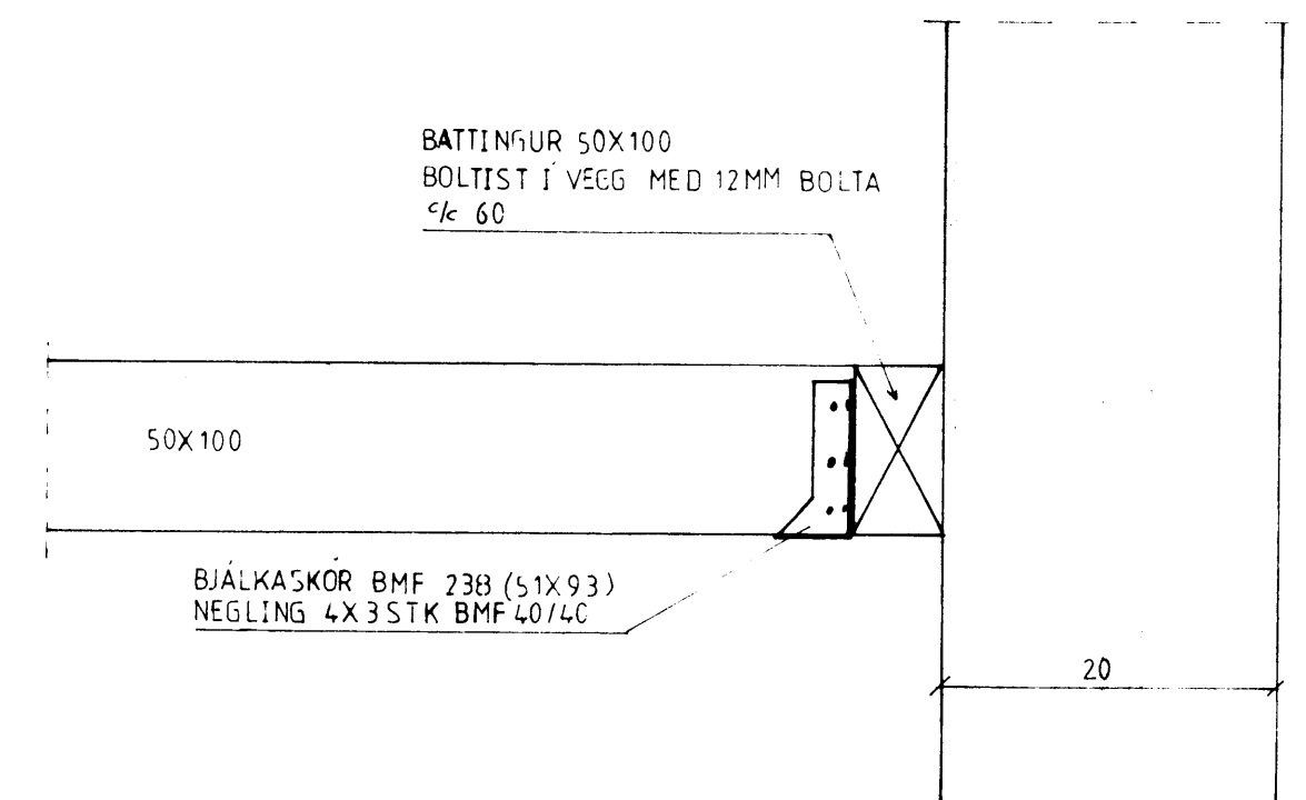
DEILI 6 1:5
