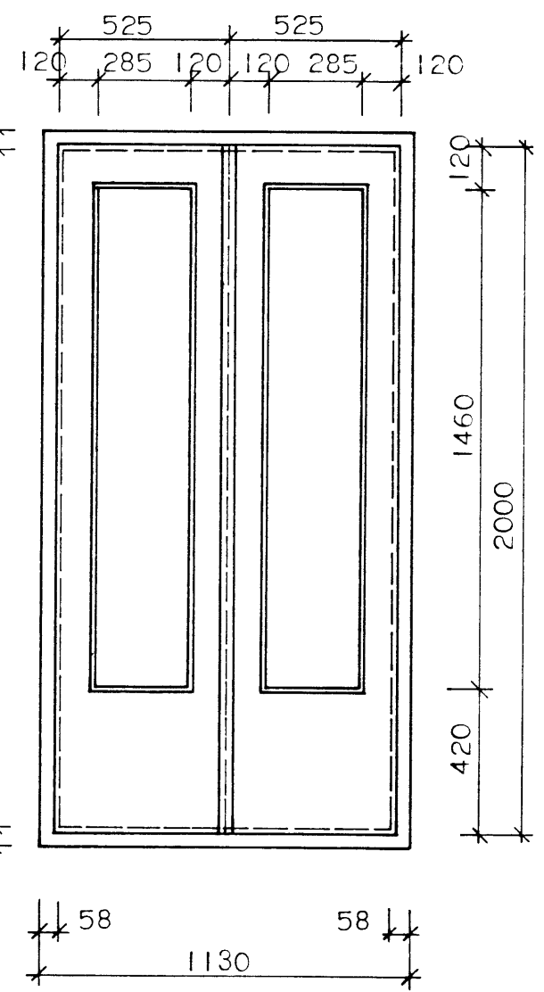
H7 1 STK GARÐHURÐ
