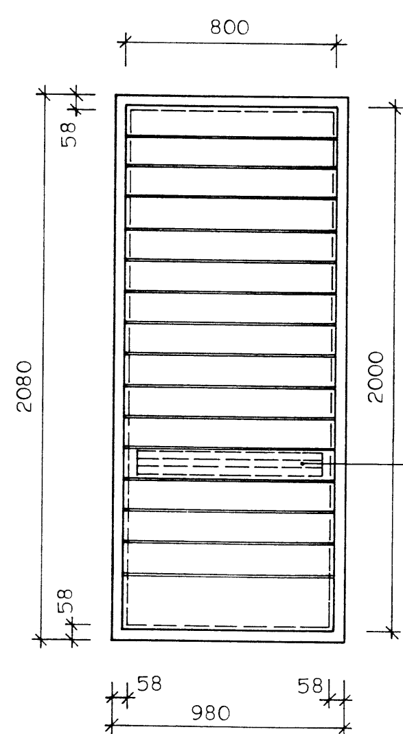
H4 2 STK SORP + INNGANGUR Í BÍLGEYMSLU
