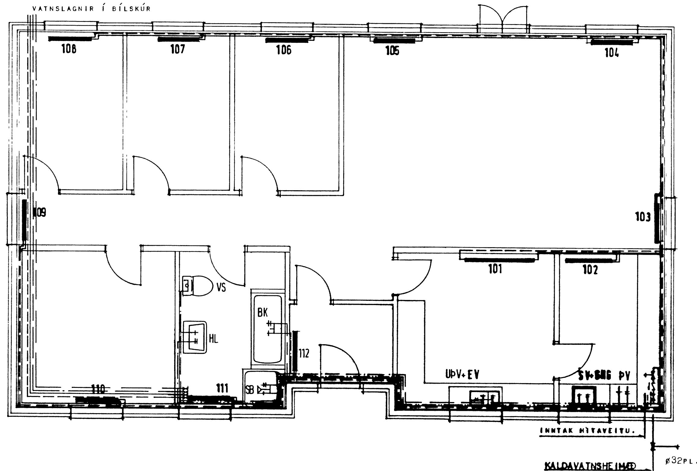
OFNASKRÁ: OFNAR VALDIR FYRIR \Delta T=40^\circ .
