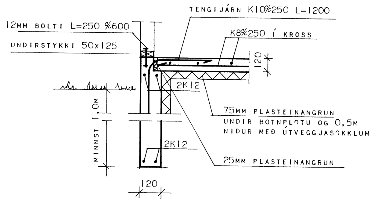
snid A-A
