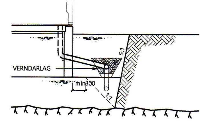
SNID VID SÖKKUL MKV. 1:50
