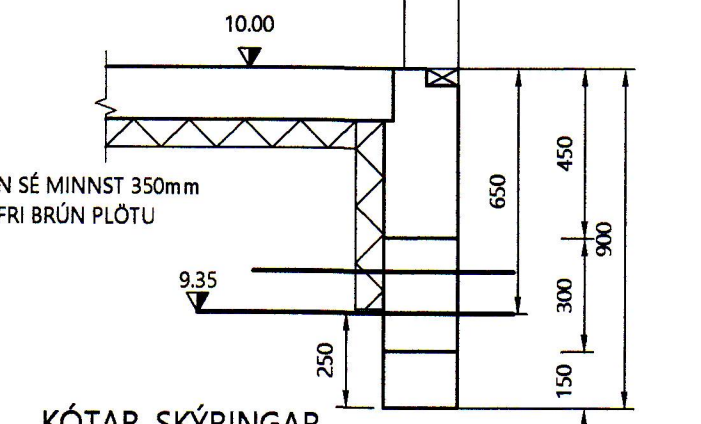
KÖTAR, SKÝRINGAR MKV. 1:20
