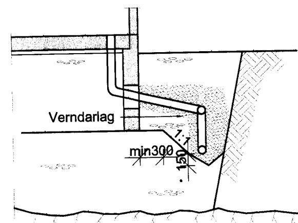
Snið við sökkul M 1:50
