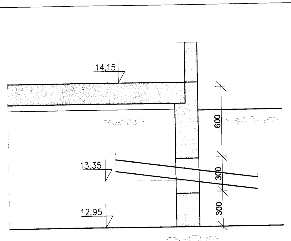
Kótar skýringar M 1:20
