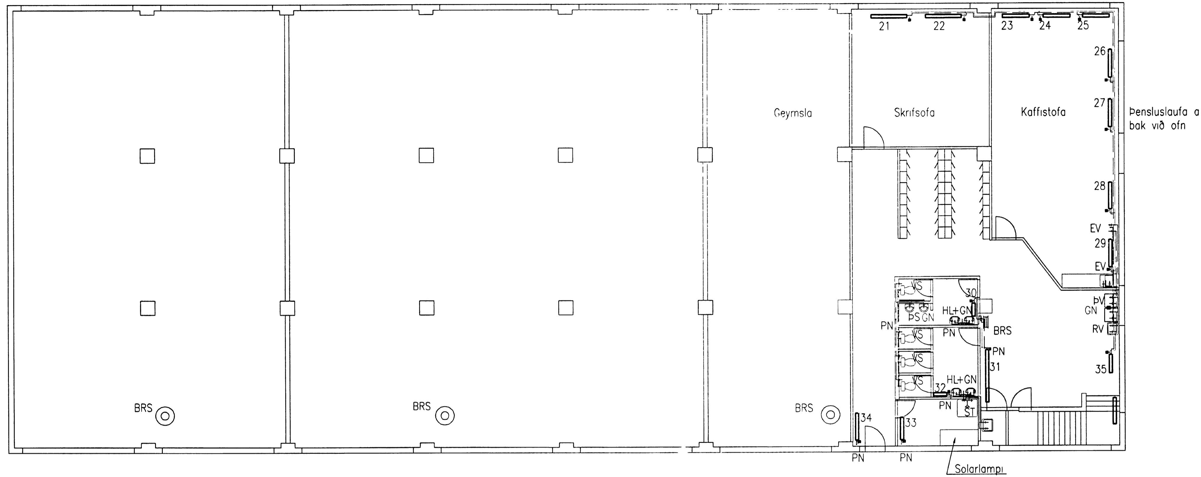
GRUNNMYND 2. HÆÐ, 1:100
