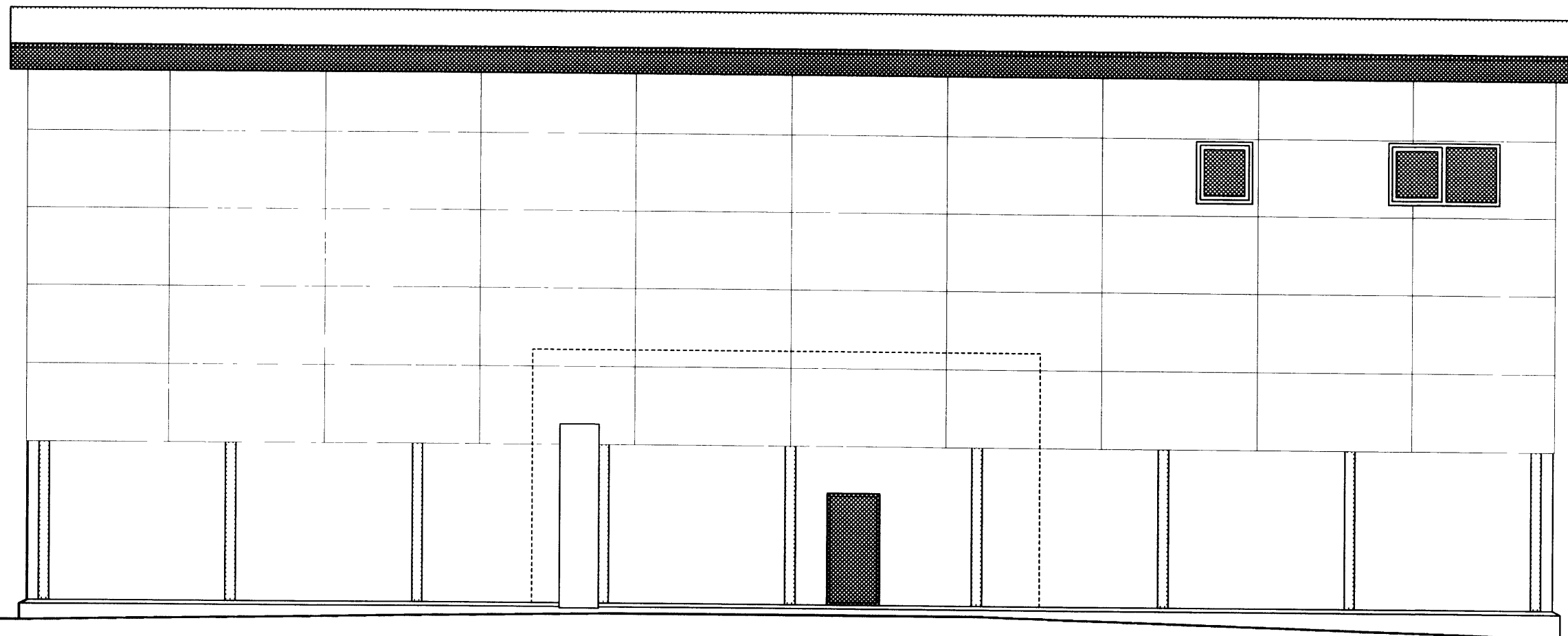
Austurhlíð, mkv 1 100
