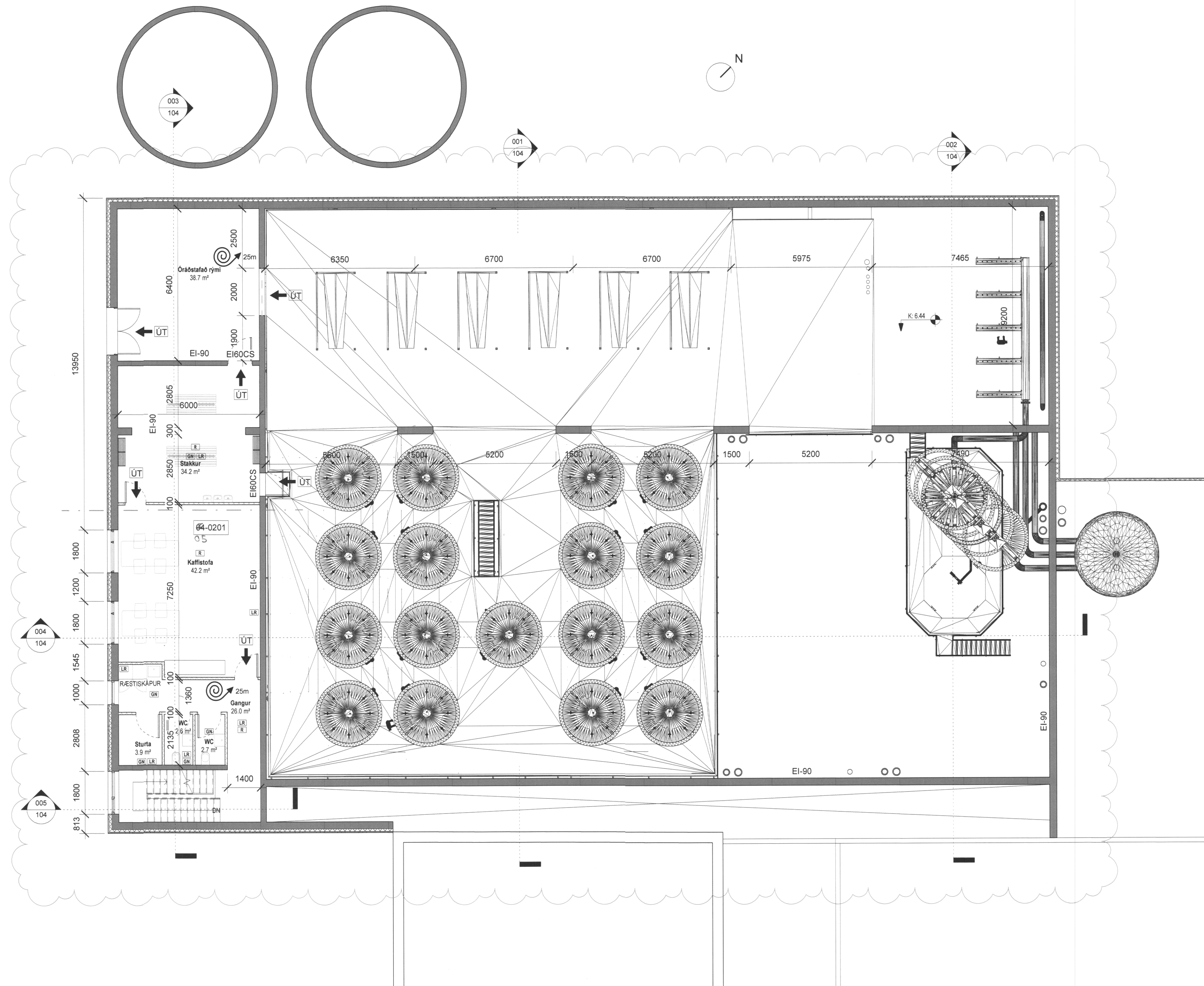
Grunnmynd 2. Hæð 1:100
