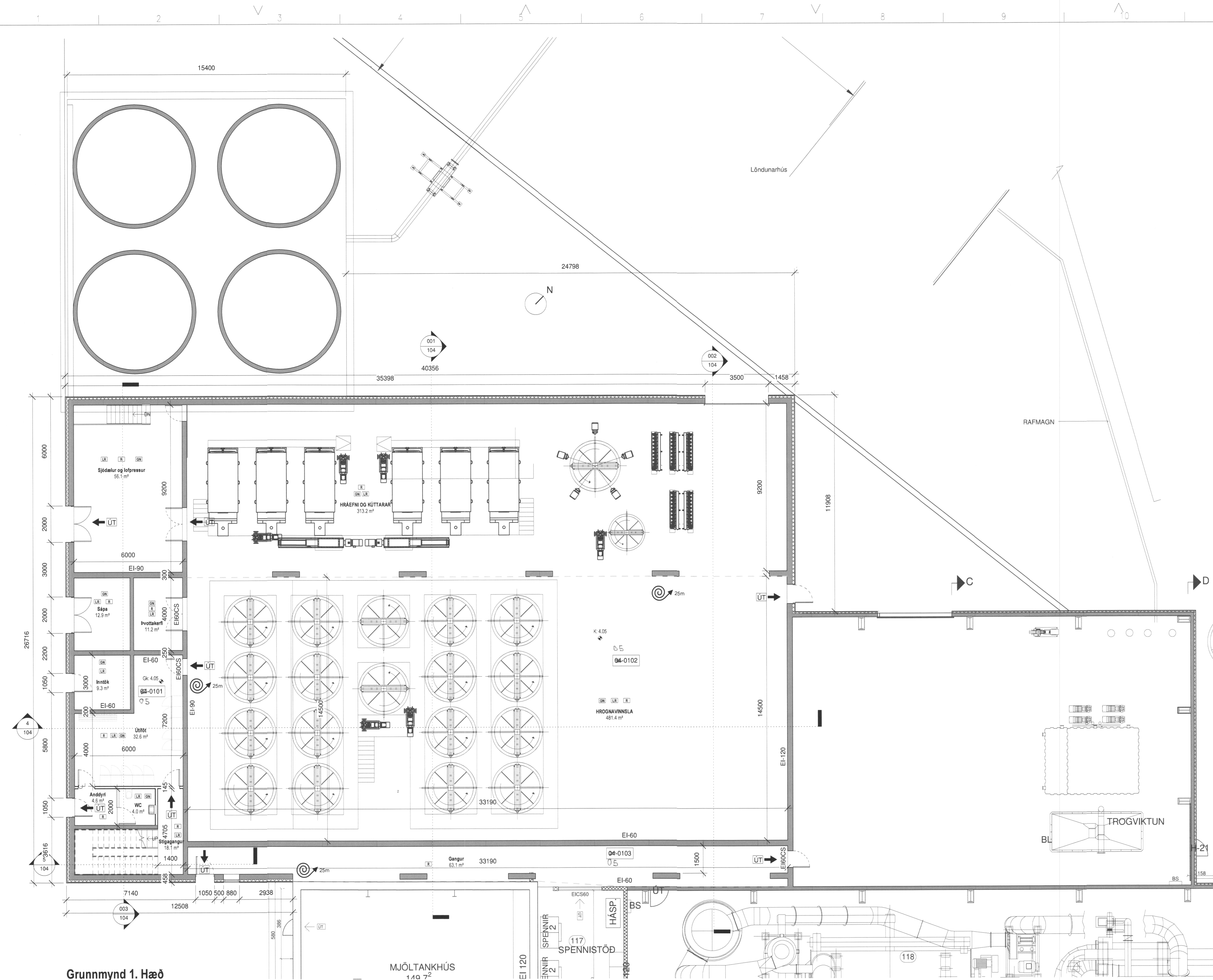
Grunnmynd 1. Hæð 1:100
