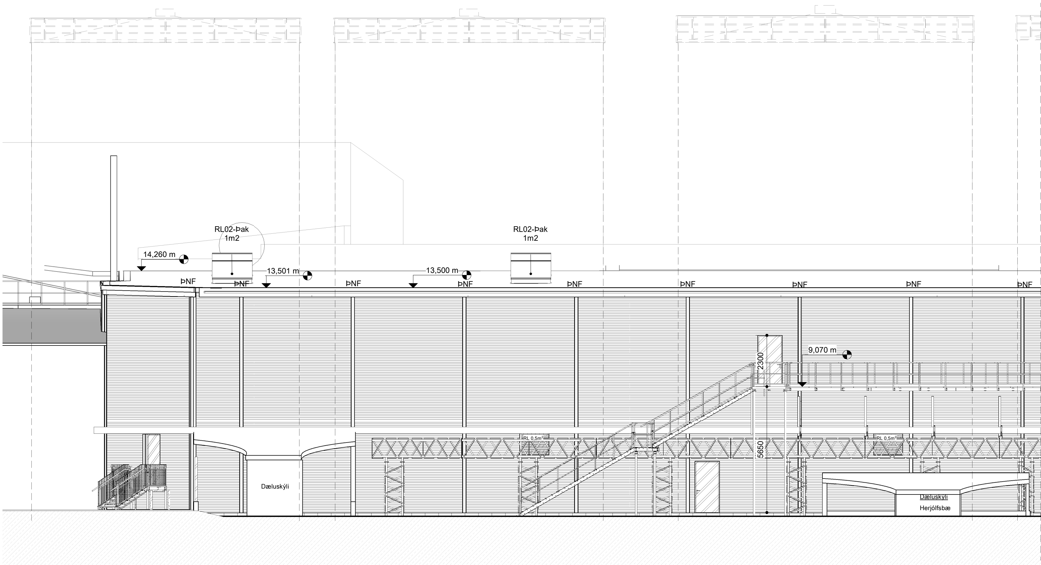
Austur. mkv: 1 : 100
