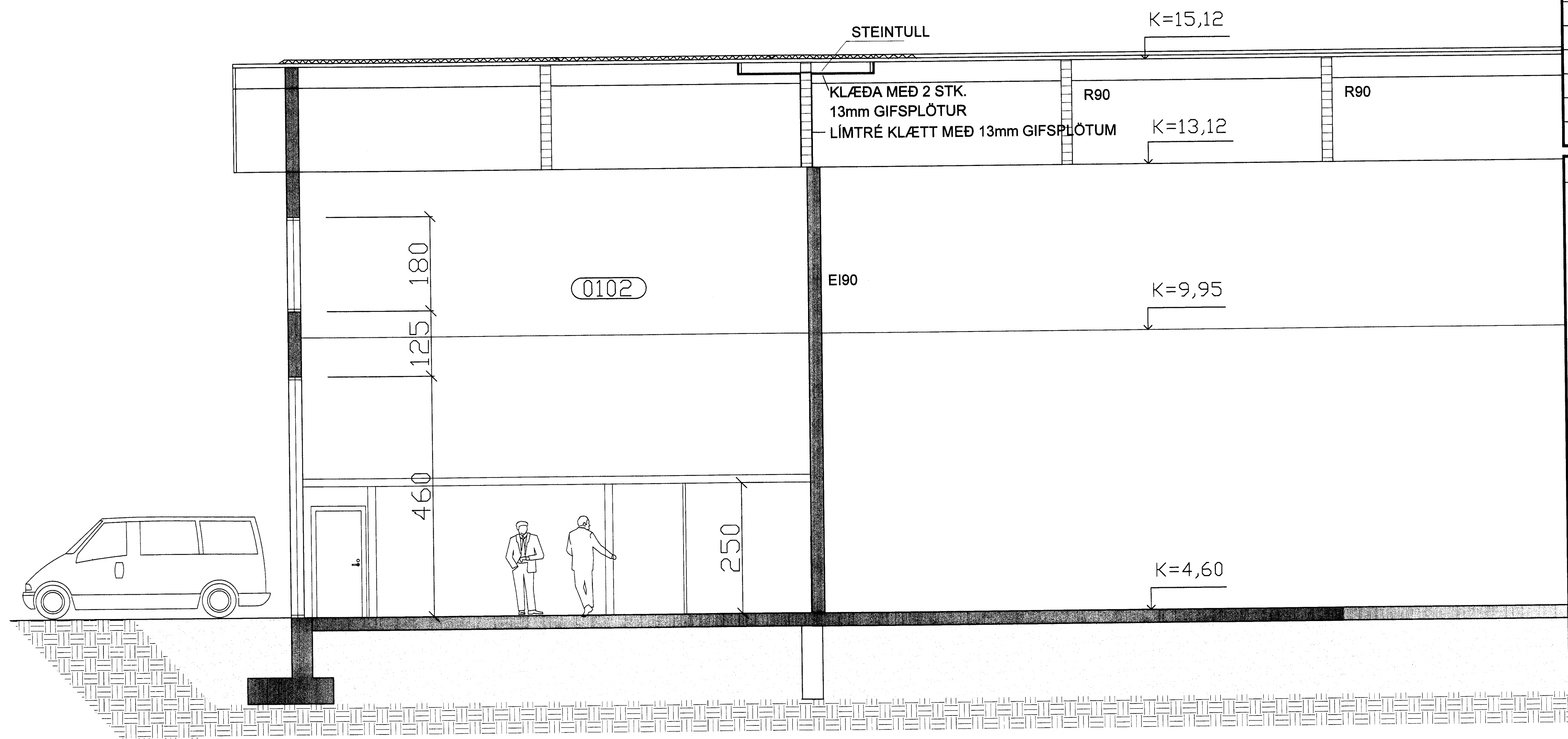
SNID A:A
