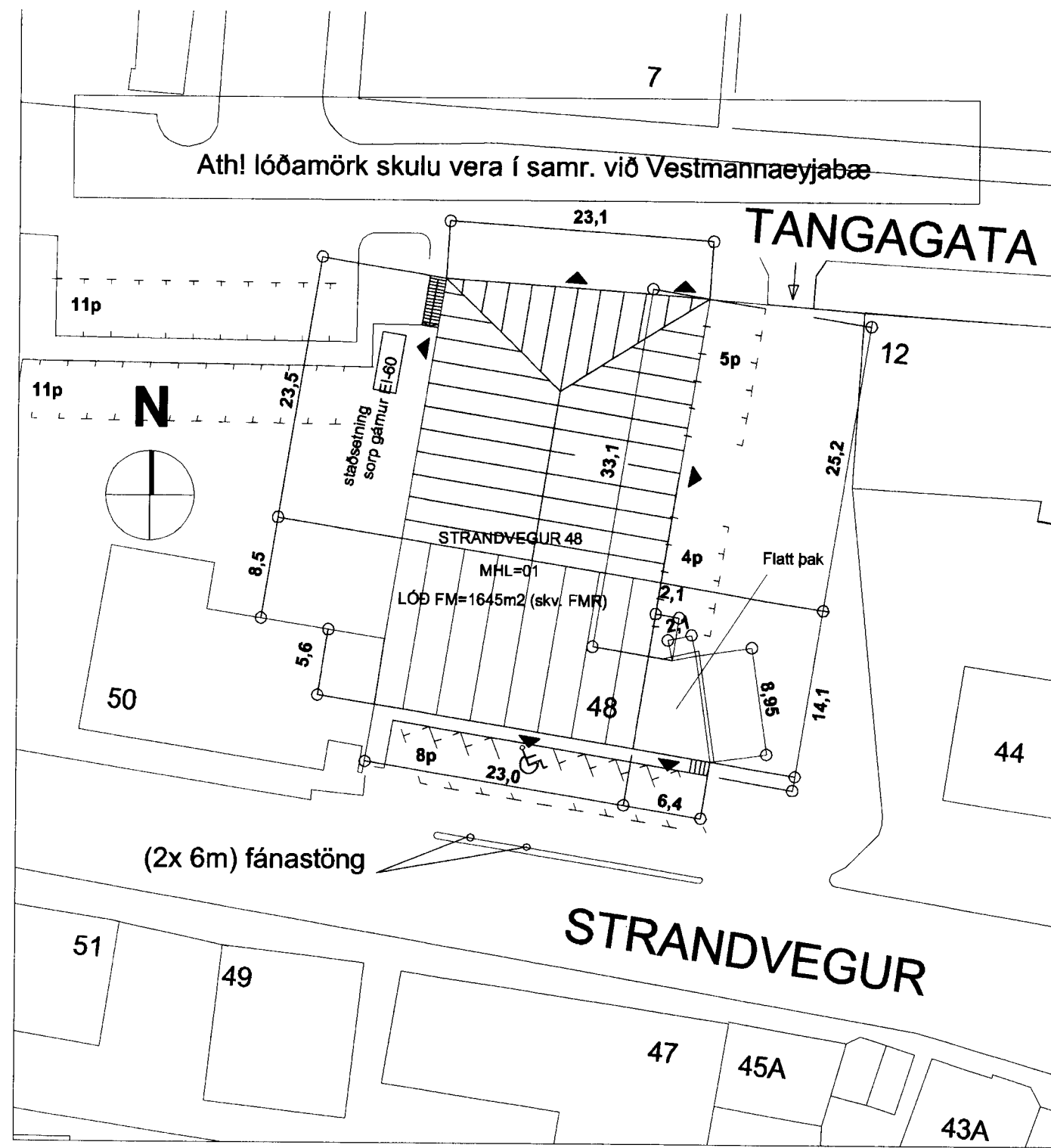
Afstöðumynd 1:500
