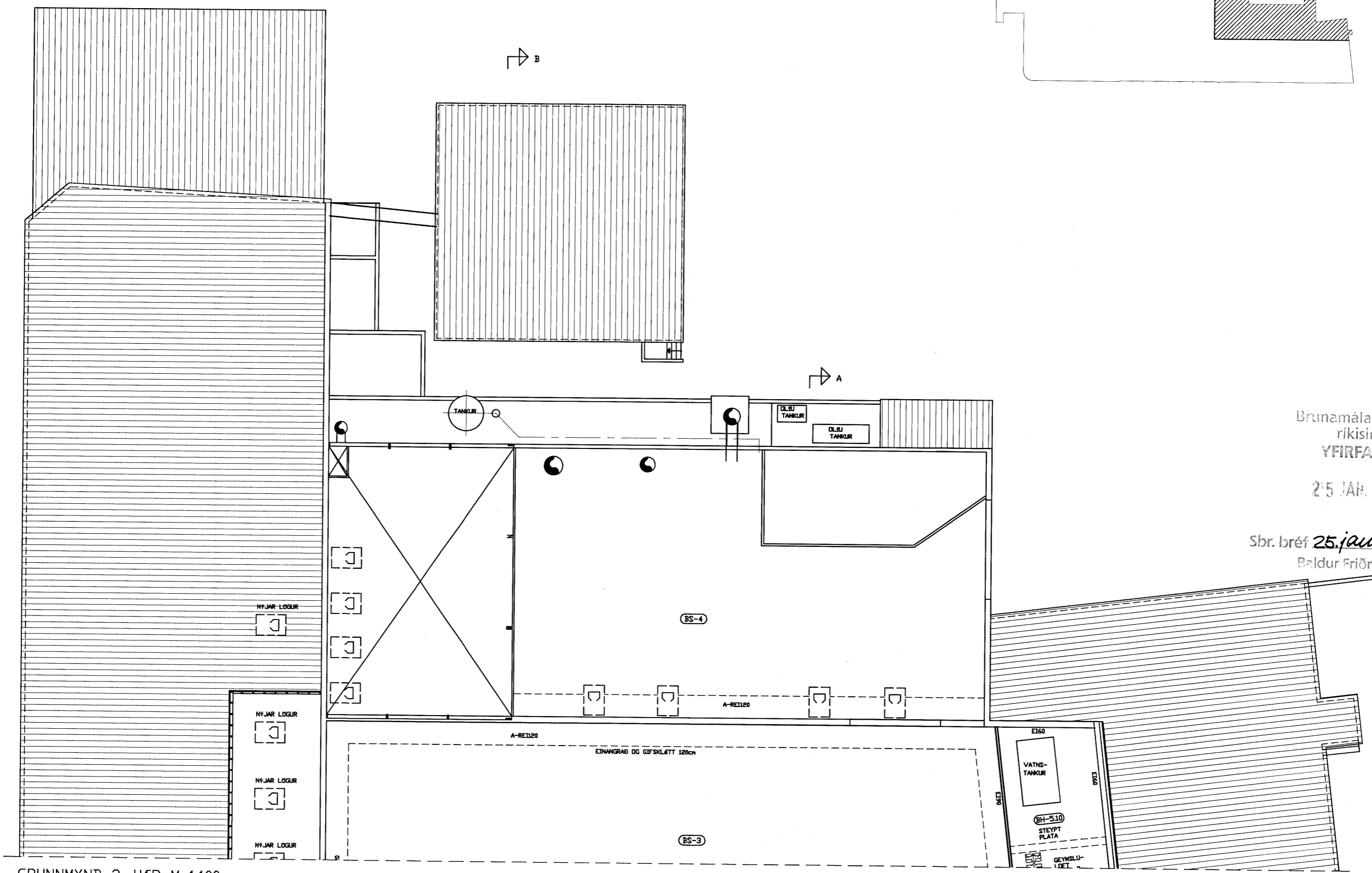
GRUNNMYND 3. HÆÐ M=1:100
