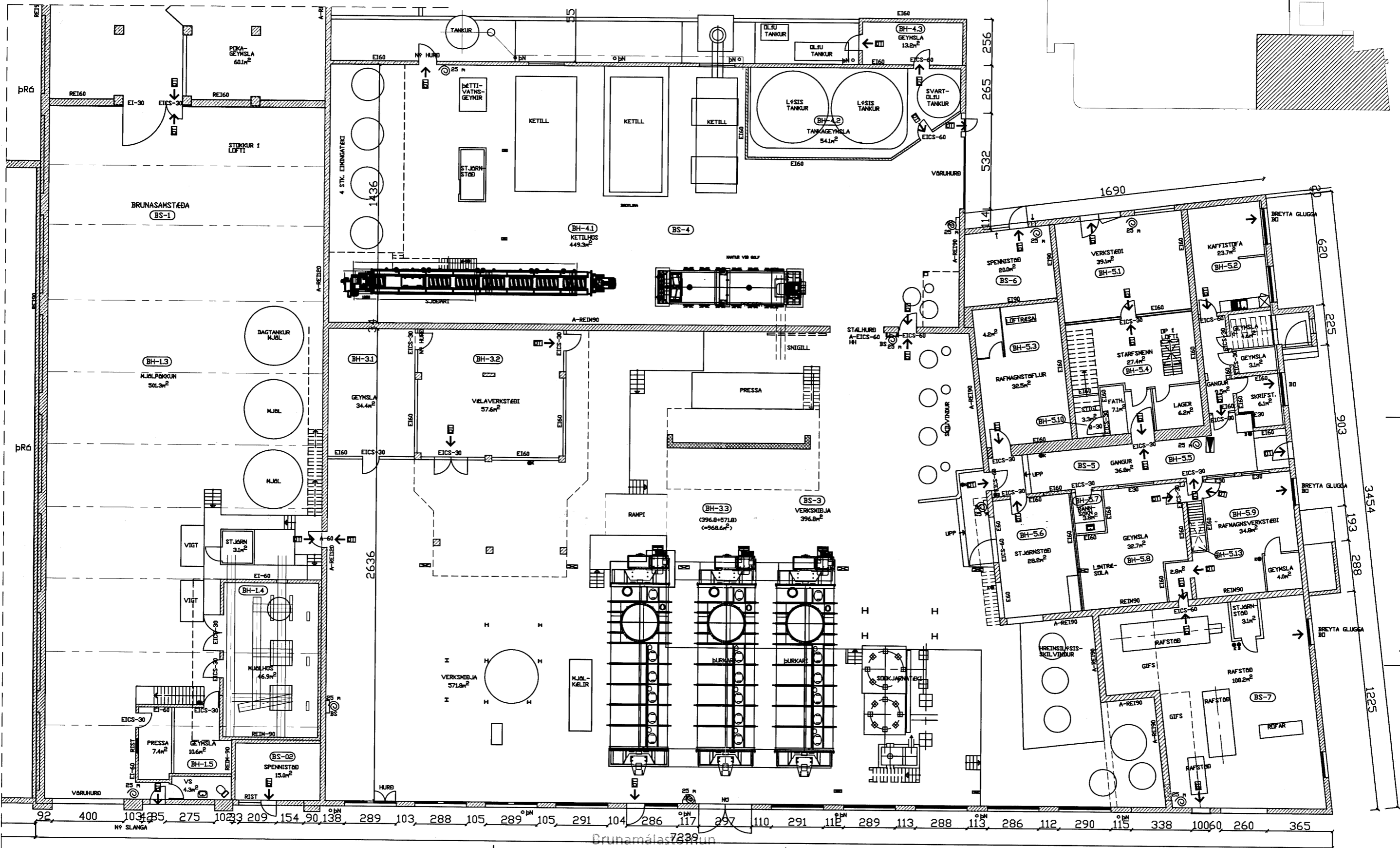
GRUNNMYND 1. HÆÐ M=1:100 SUÐURENDI VESTUR
