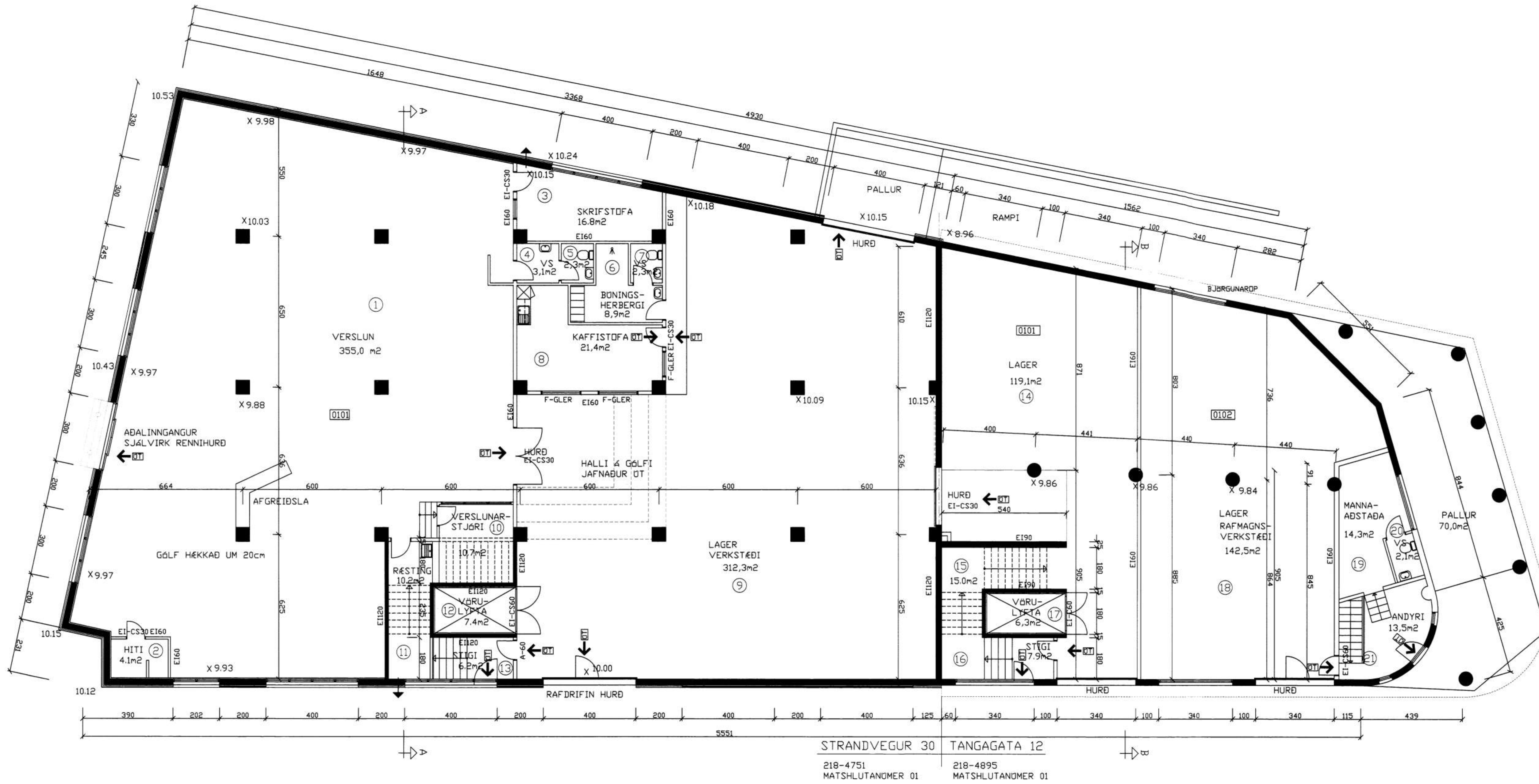
GRUNNMYND 1. HÆÐ
