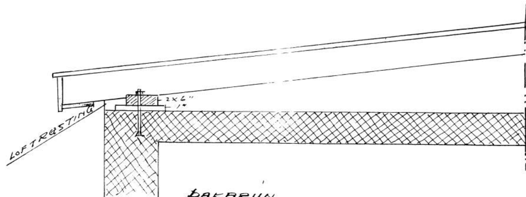
ÞAKBRUN 1:10
