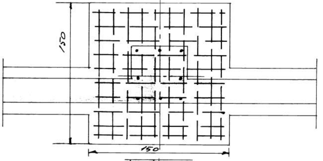
VEGGJÚLUR: UNDIRSTÖÐUR 1:20
