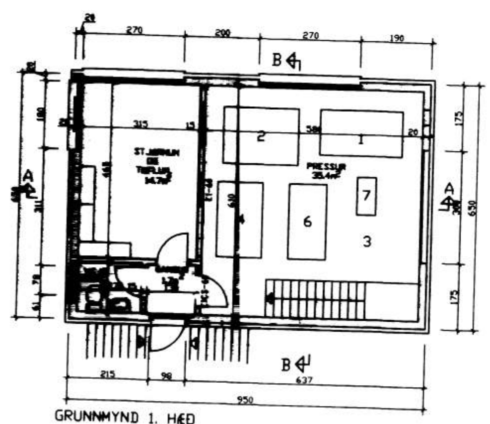
GRUNNMYND 1. HÆÐ
