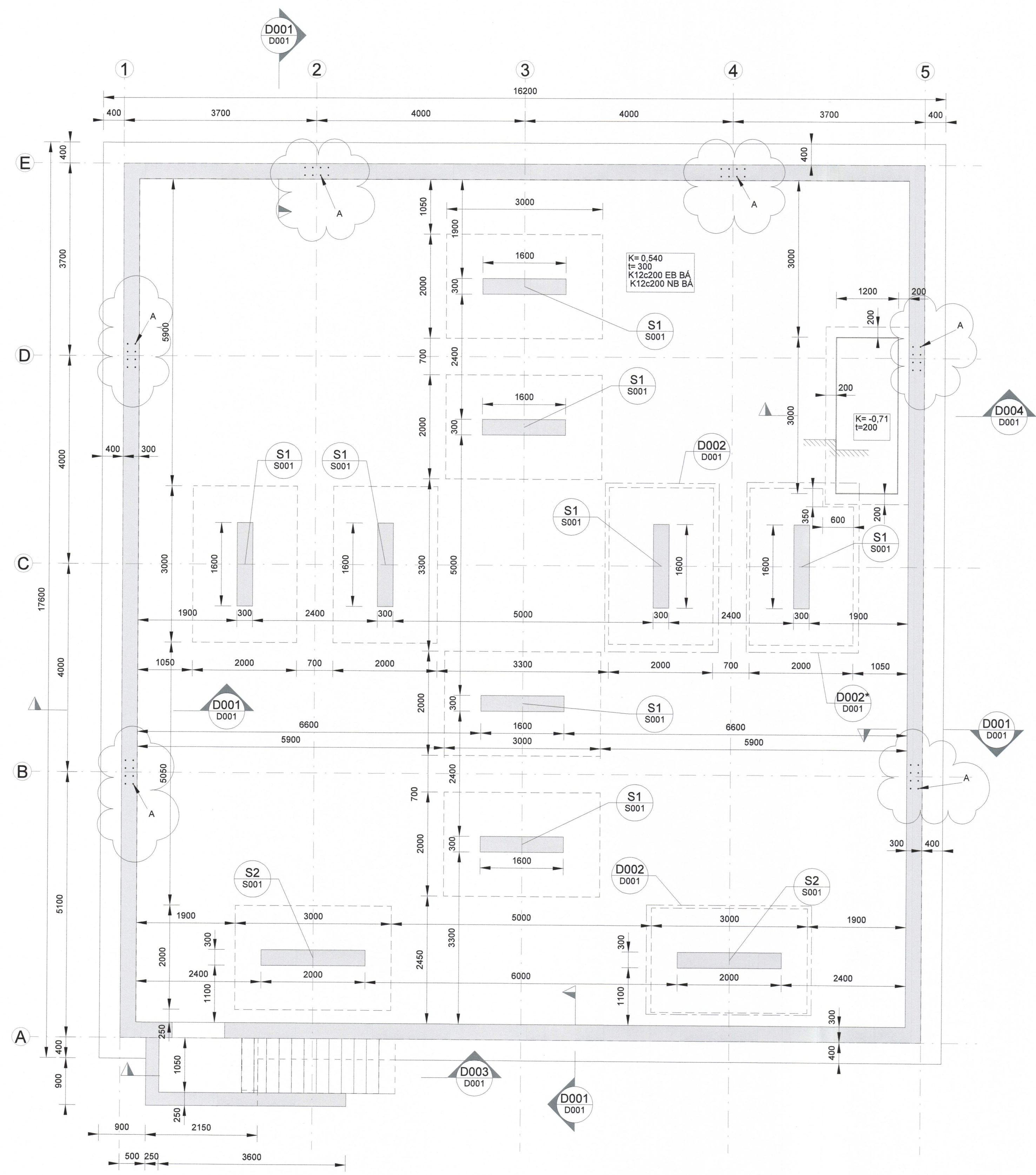
GRUNNMYND 1:50
