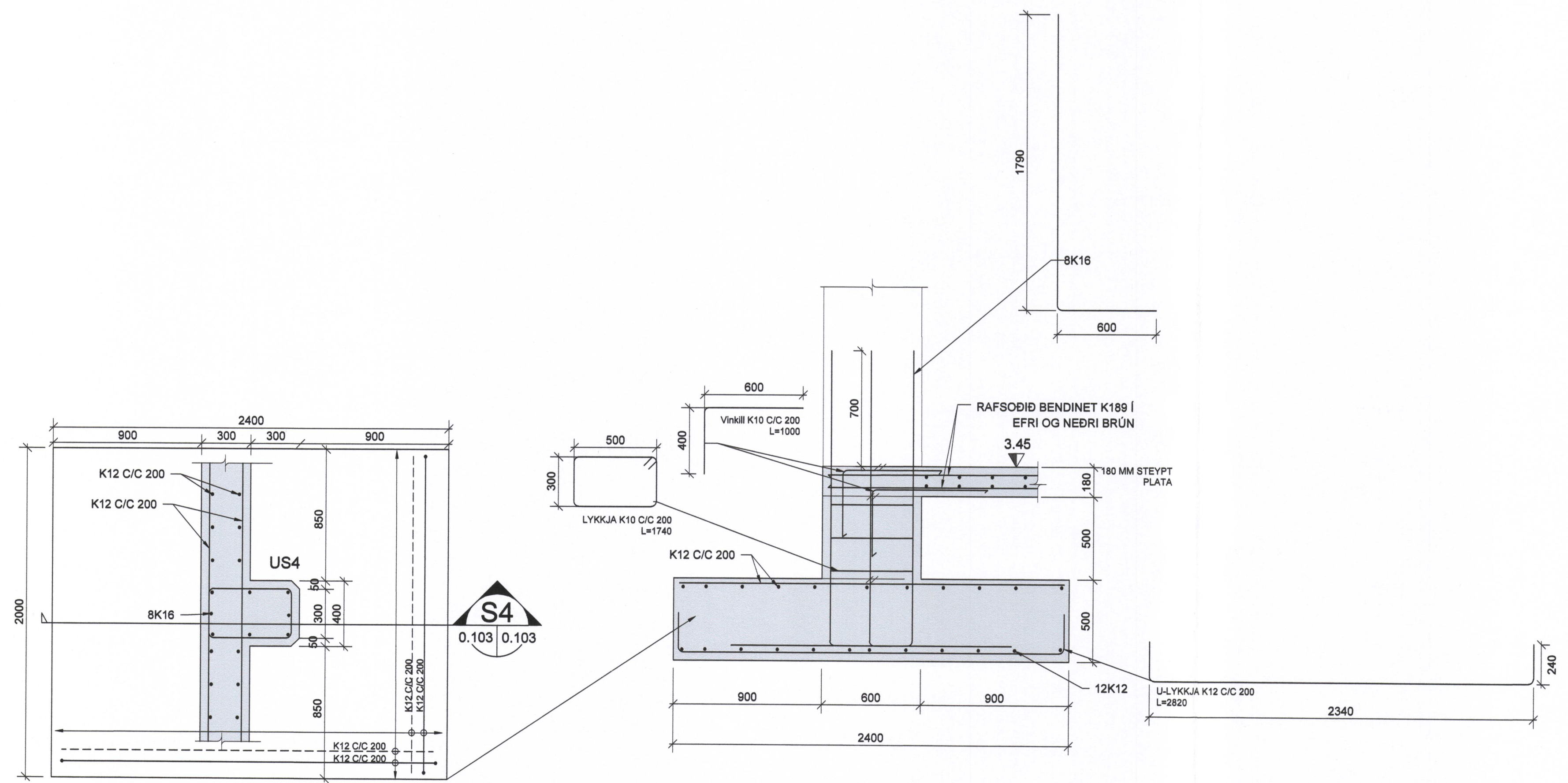
S4 SNID 0.103 0.103 1:20
