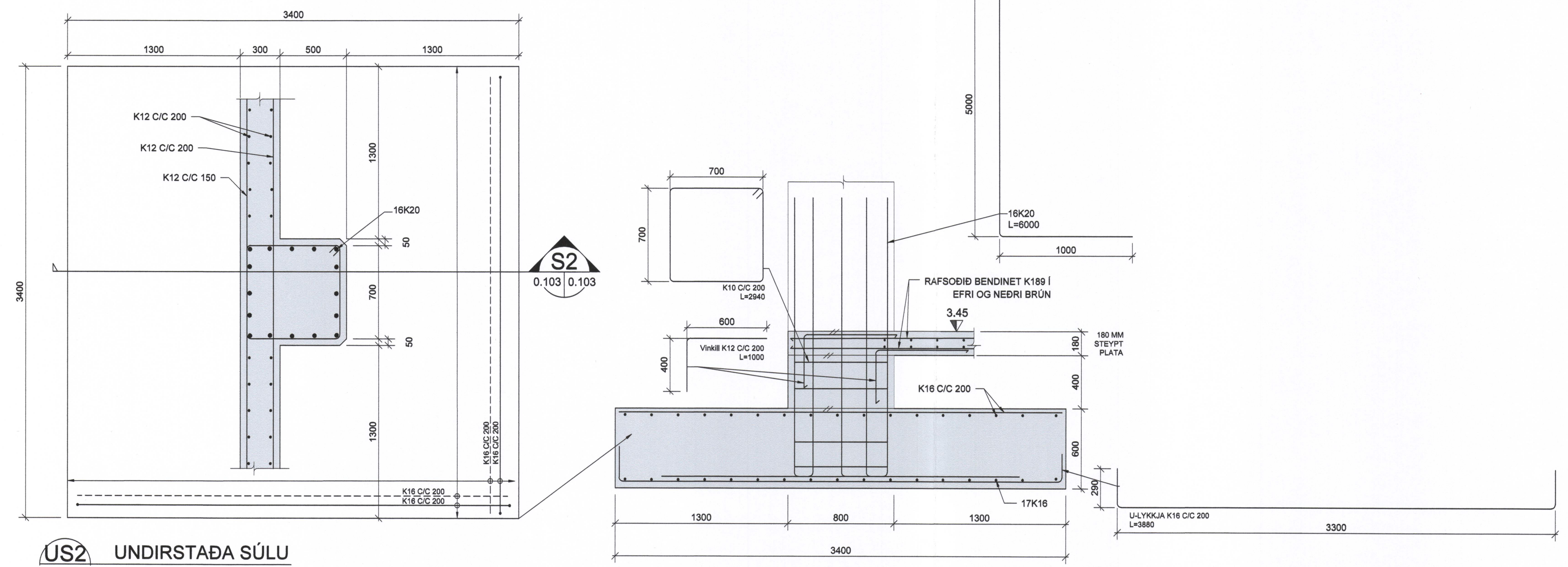
S2 SNID 0.103 0.103 1:20
