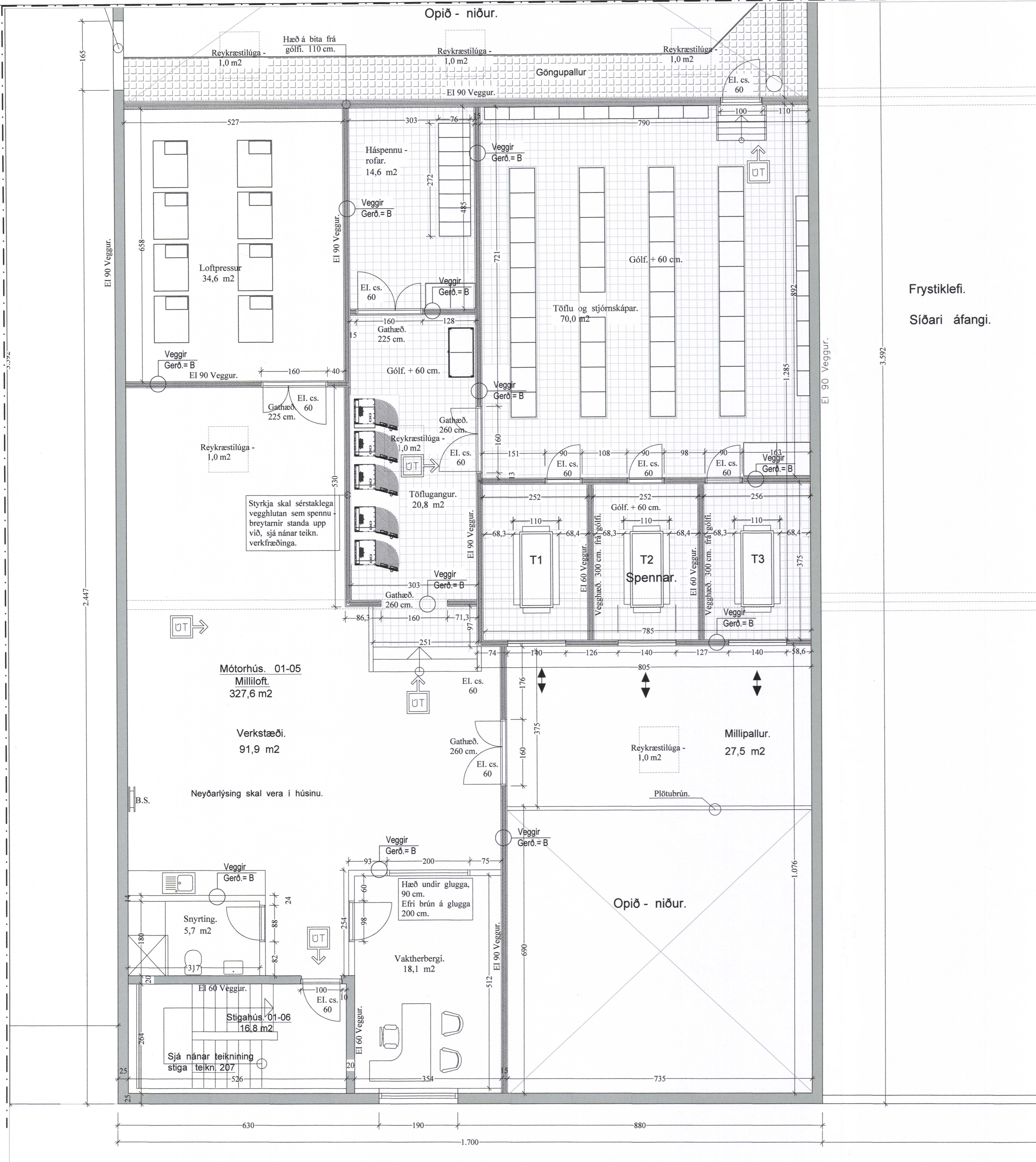
Grunnmynd. 2. Hæð 1:50 Mótórhús.
