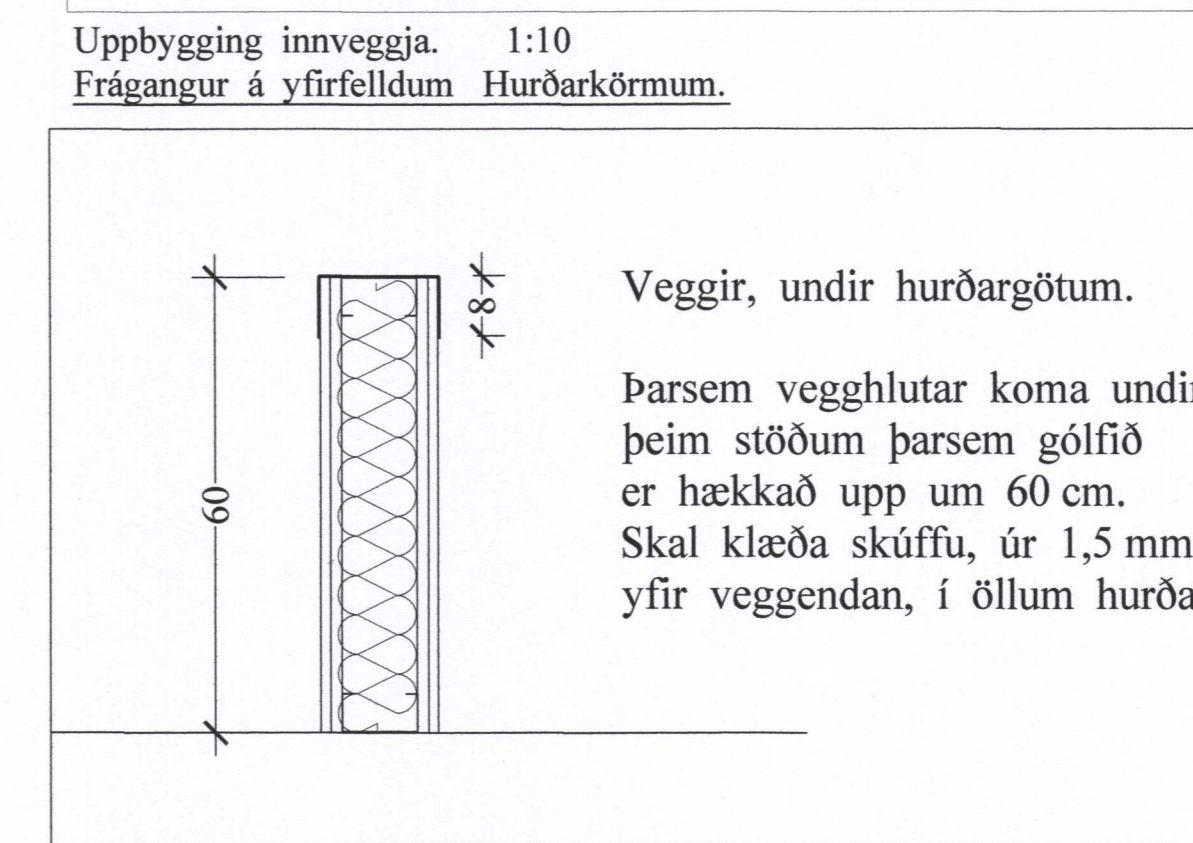
Frágangur veggja undir hurðargötum. 1:10 Mótórhús.
