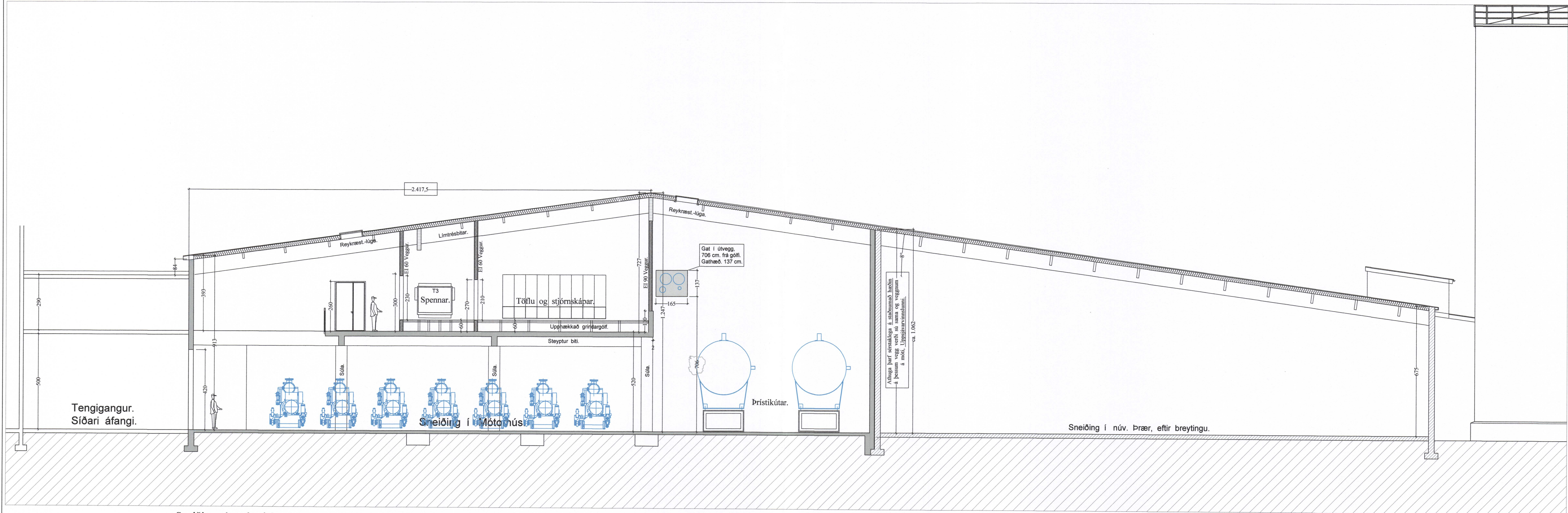
Sneiðing í mótórhús og núv. Prær. 1:100
