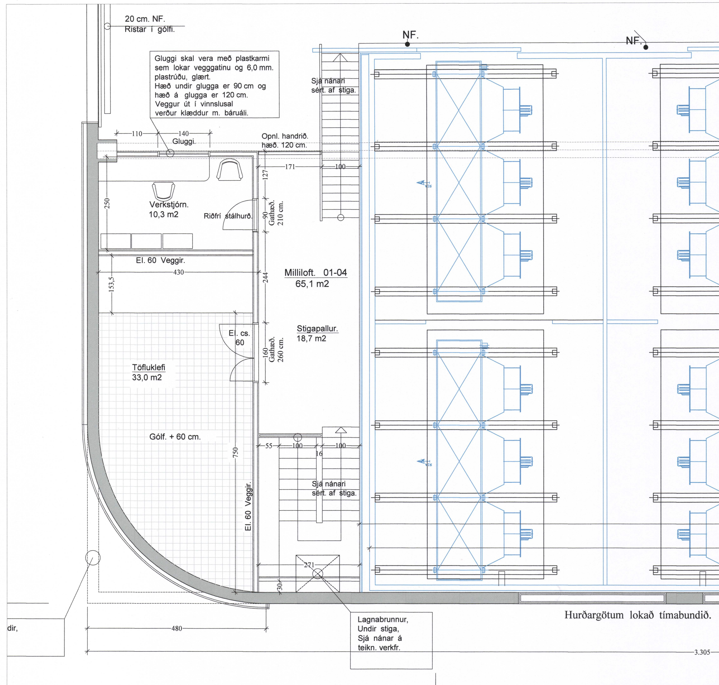
Grunnmynd Milliloft. Hlutamynd. 1:50
