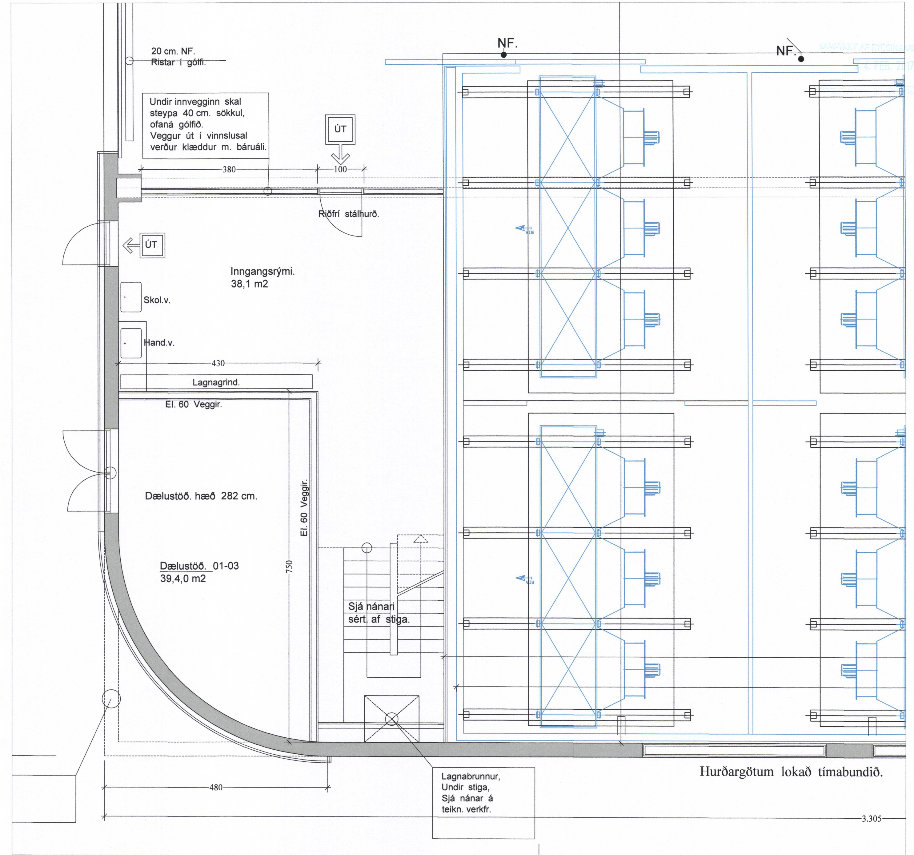
Grunnmynd Jarðhæð. Hlutamynd. 1:50
