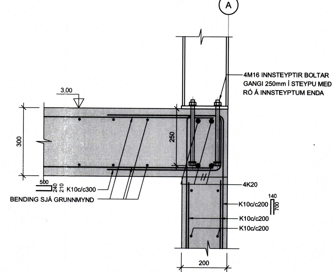
SNID A-A FYRIR IF5 1:10
