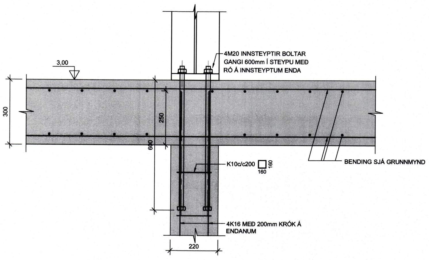
SNID A-A FYRIR IF4 1:10
