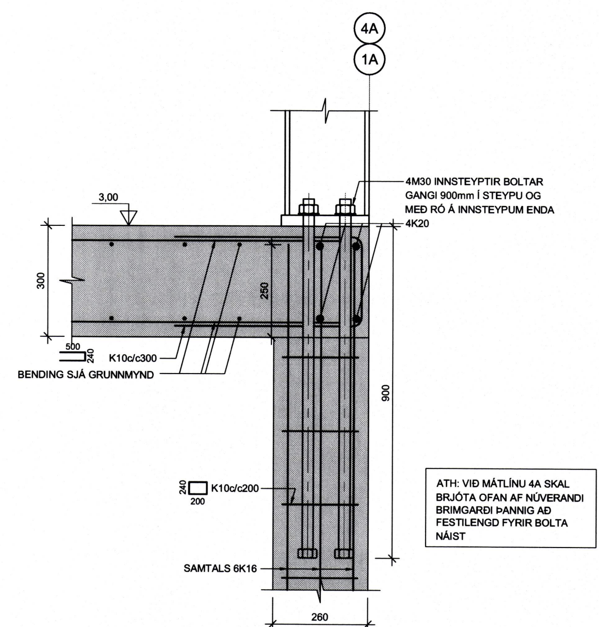
SNID A-A FYRIR IF3 1:10
