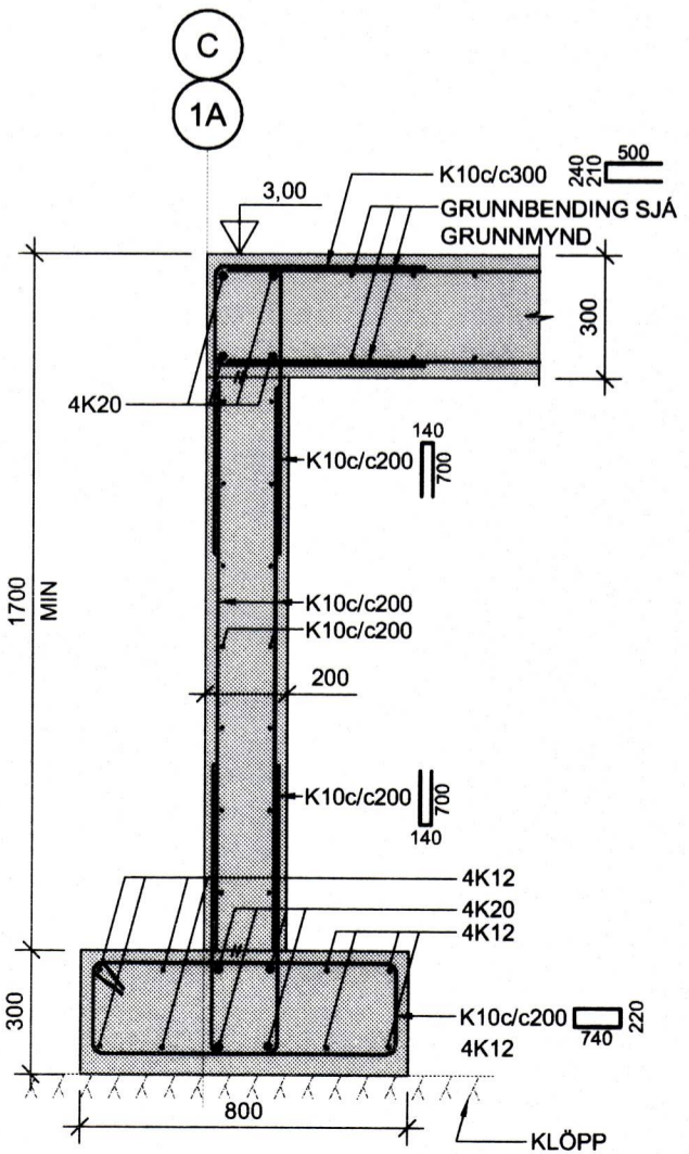
1 SNID 1:20 B-100
