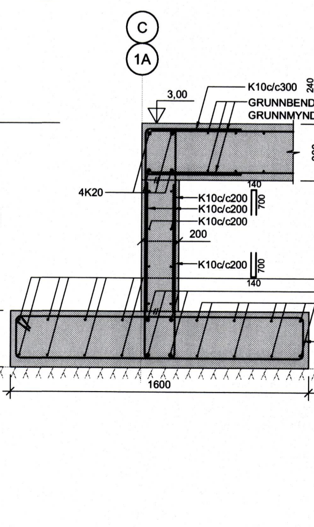
5 SNID 1:20 B-100
