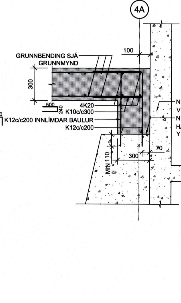
3 SNID 1:20 B-100
