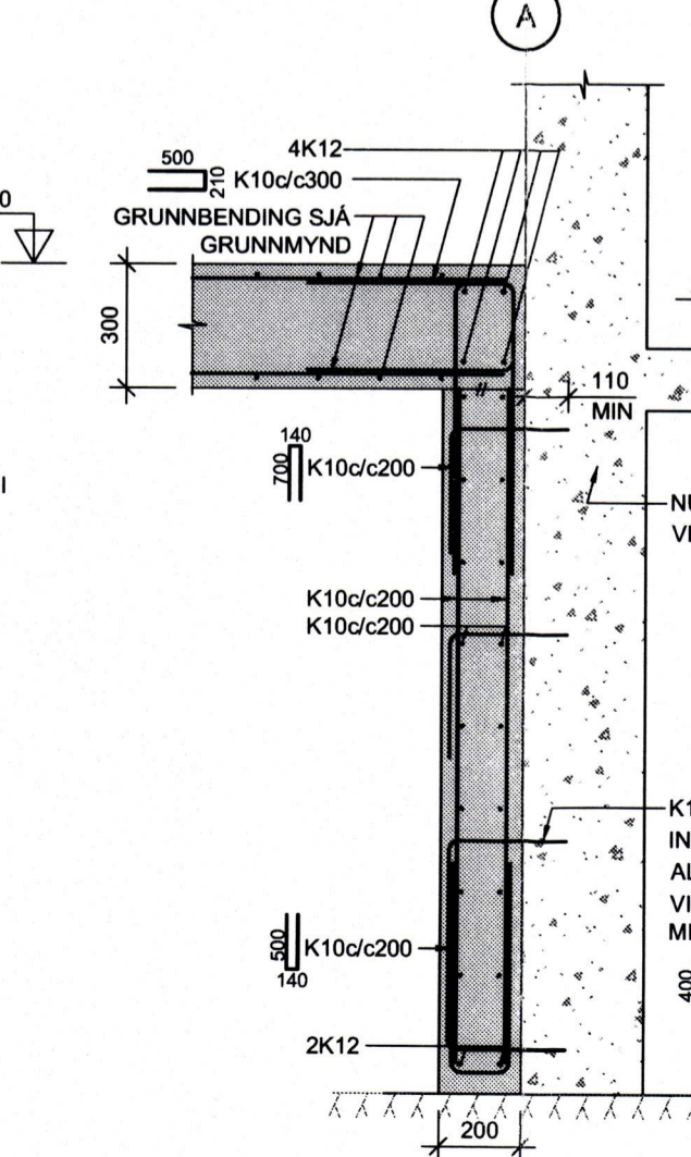
4 SNID 1:20 B-100
