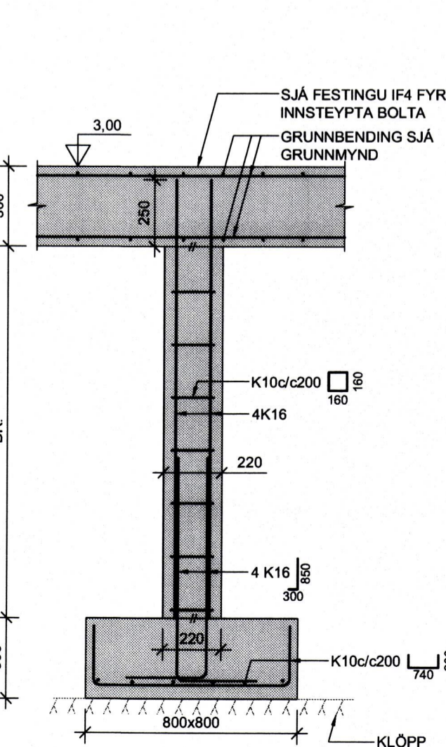
2 SNID 1:20 B-100
