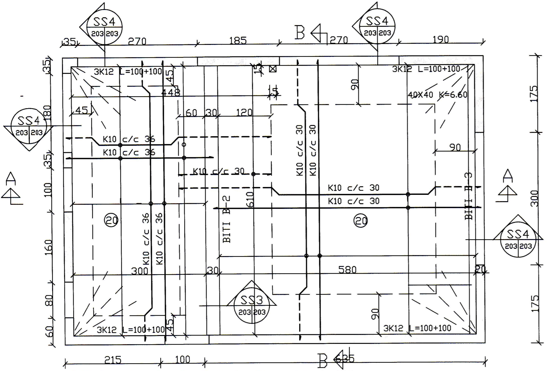
GRUNNMYND STEYPT PLATA þAK
