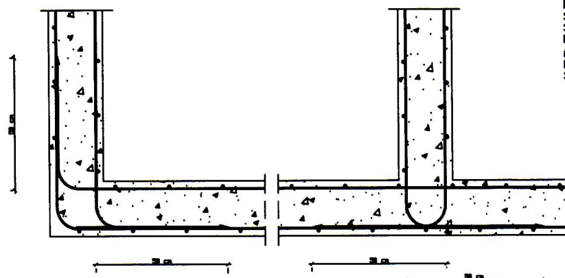
LAGNING LARÉTTRA JÄRNA UM HÖRN Í VEGGJUM M=1:10
