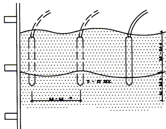
SKÝRINGAMYND: TITRUN STEYPU Í VEGG
