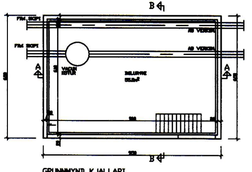
GRUNNMYND KJALLARI
