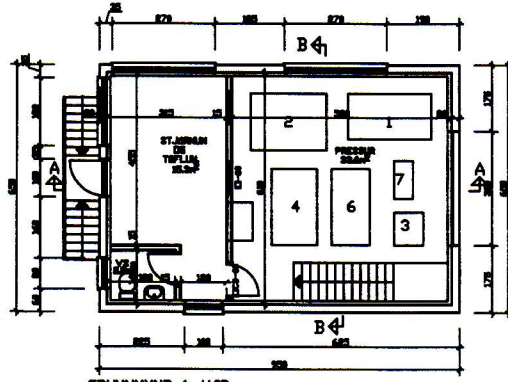
GRUNNMYND 1. HED
