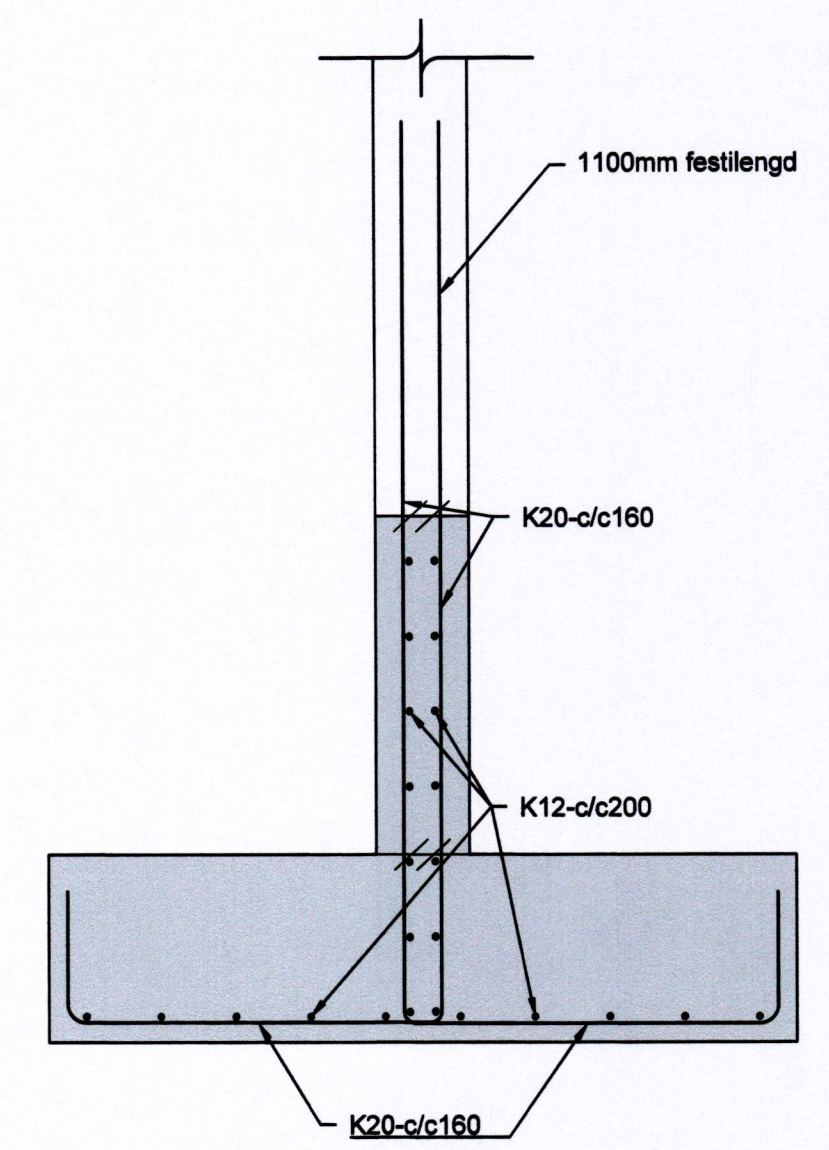
2 SNID 0120 0160 1:20
