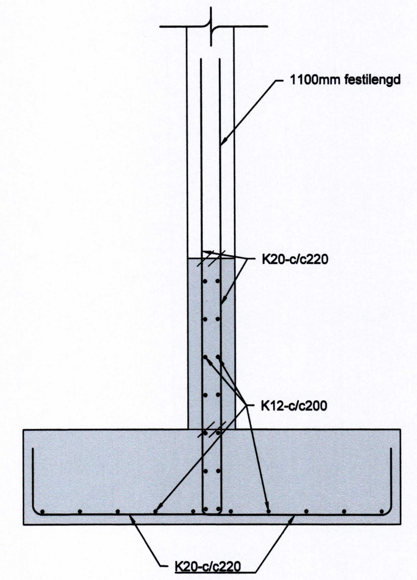
3 SNID 0120 0160 1:20
