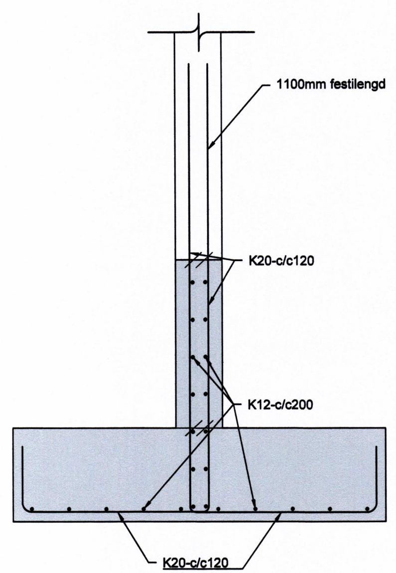
1 SNID 0120 0160 1:20
