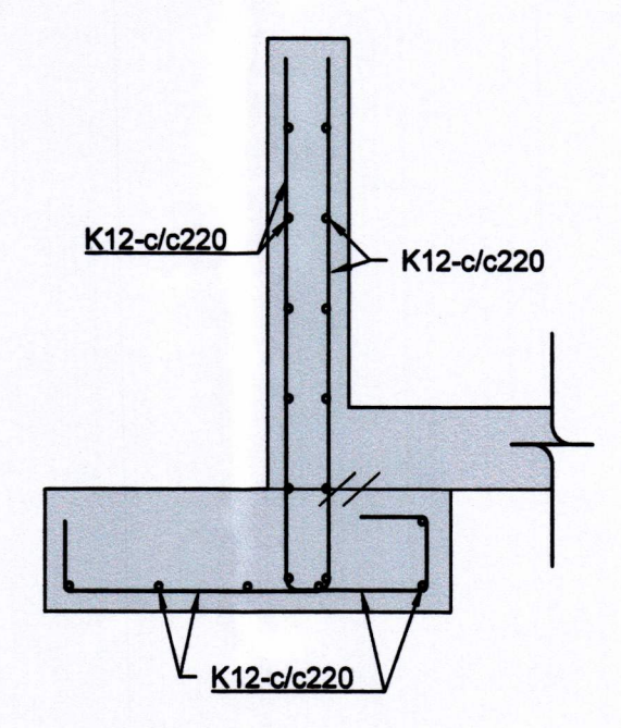
4 SNID 0120 0160 1:20
