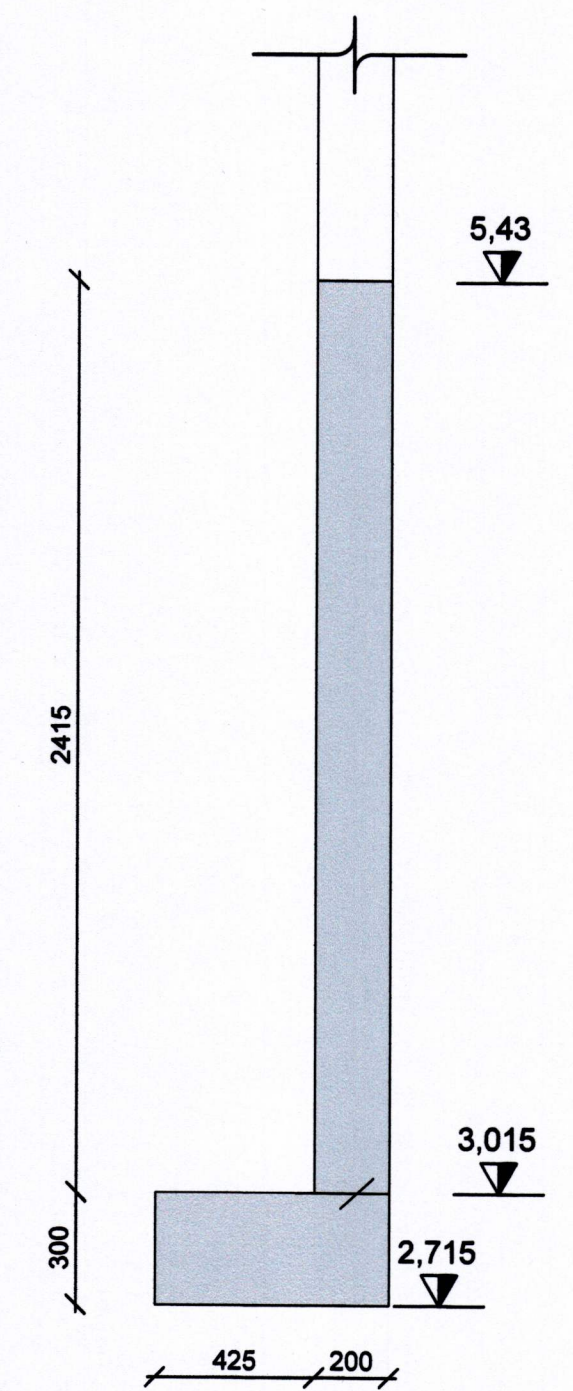
5 SNIÐ 0130 0150 1:20
