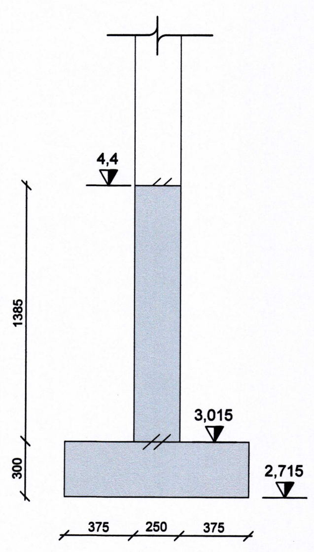
2 SNIÐ 0130 0150 1:20
