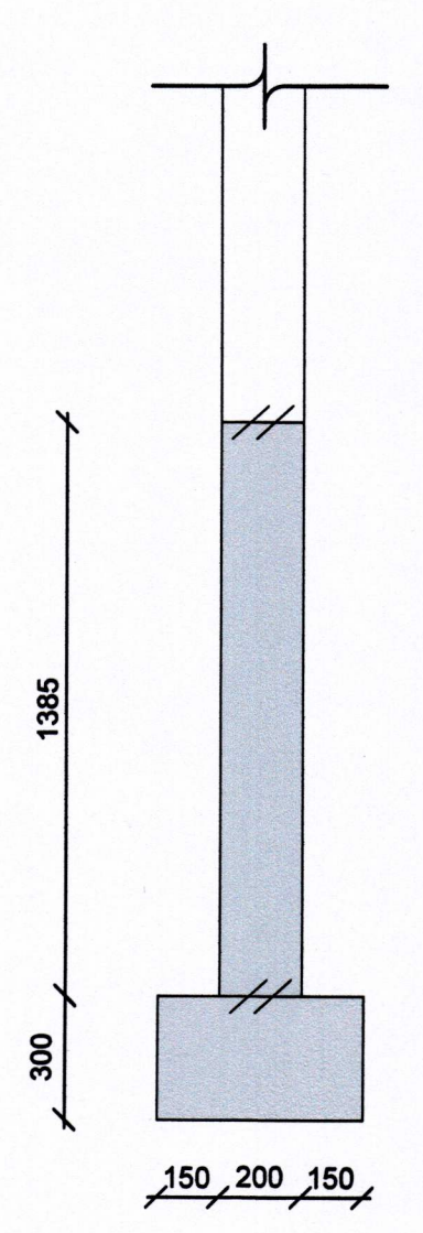
3 SNIÐ 0130 0150 1:20
