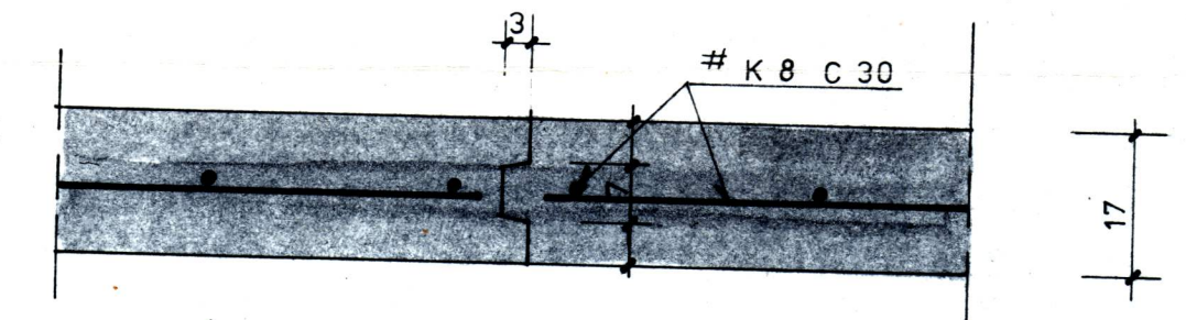
SNID Í PLÖTUSAMSKEYTI. M = 1:10
