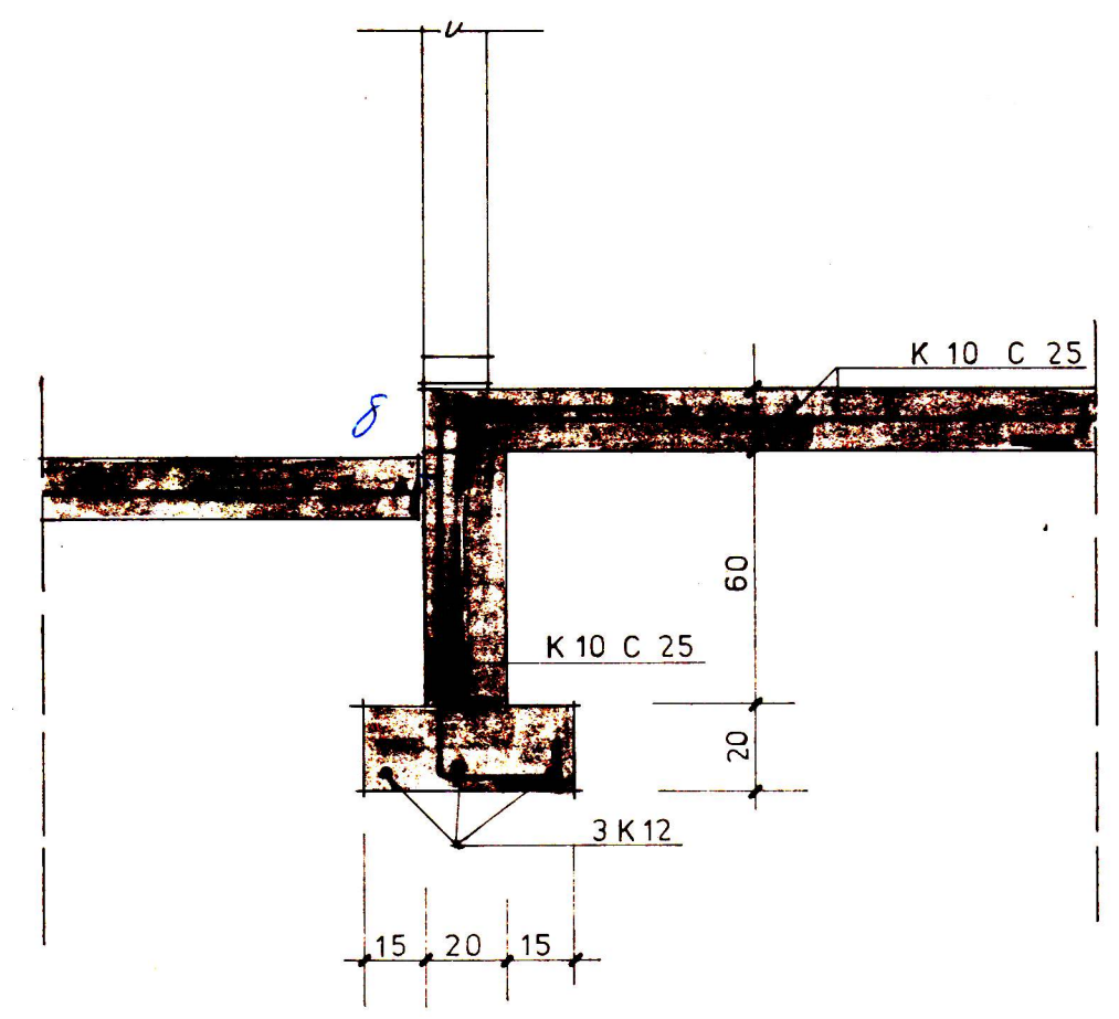
SNID Í UNDIRSTÖÐUR, A-A M=1:20
