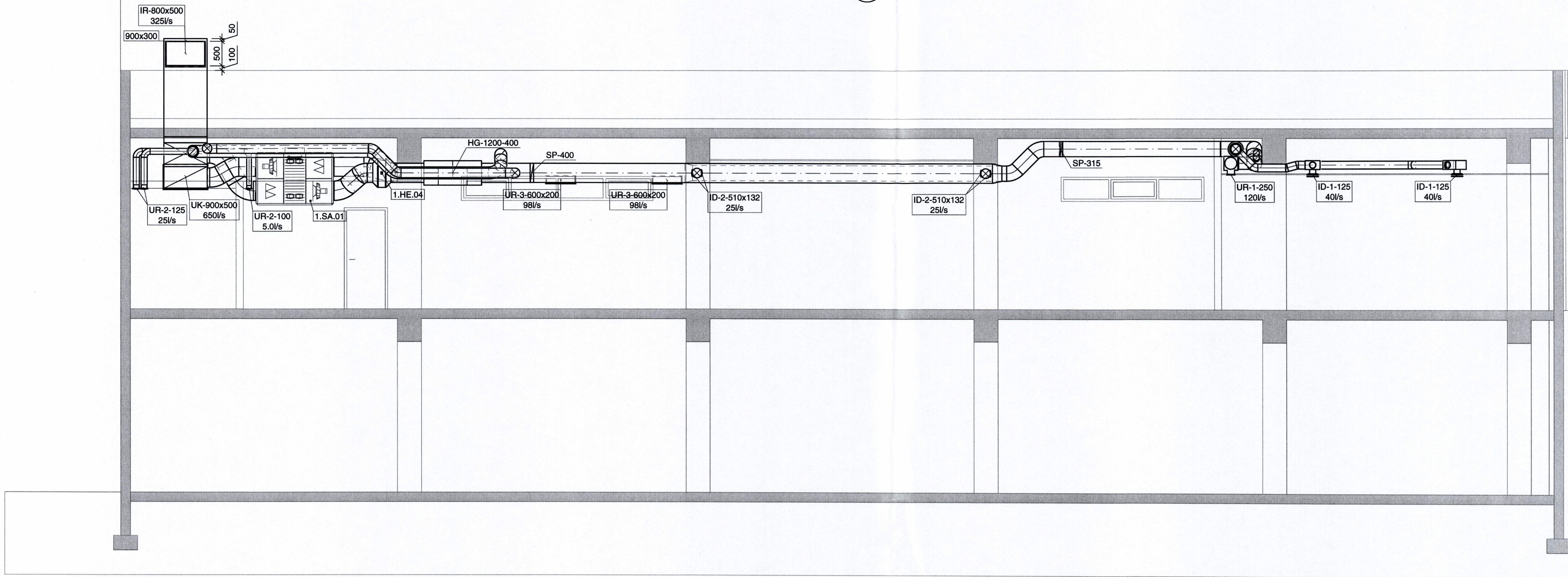
A SNIÐ L-501 1:50
