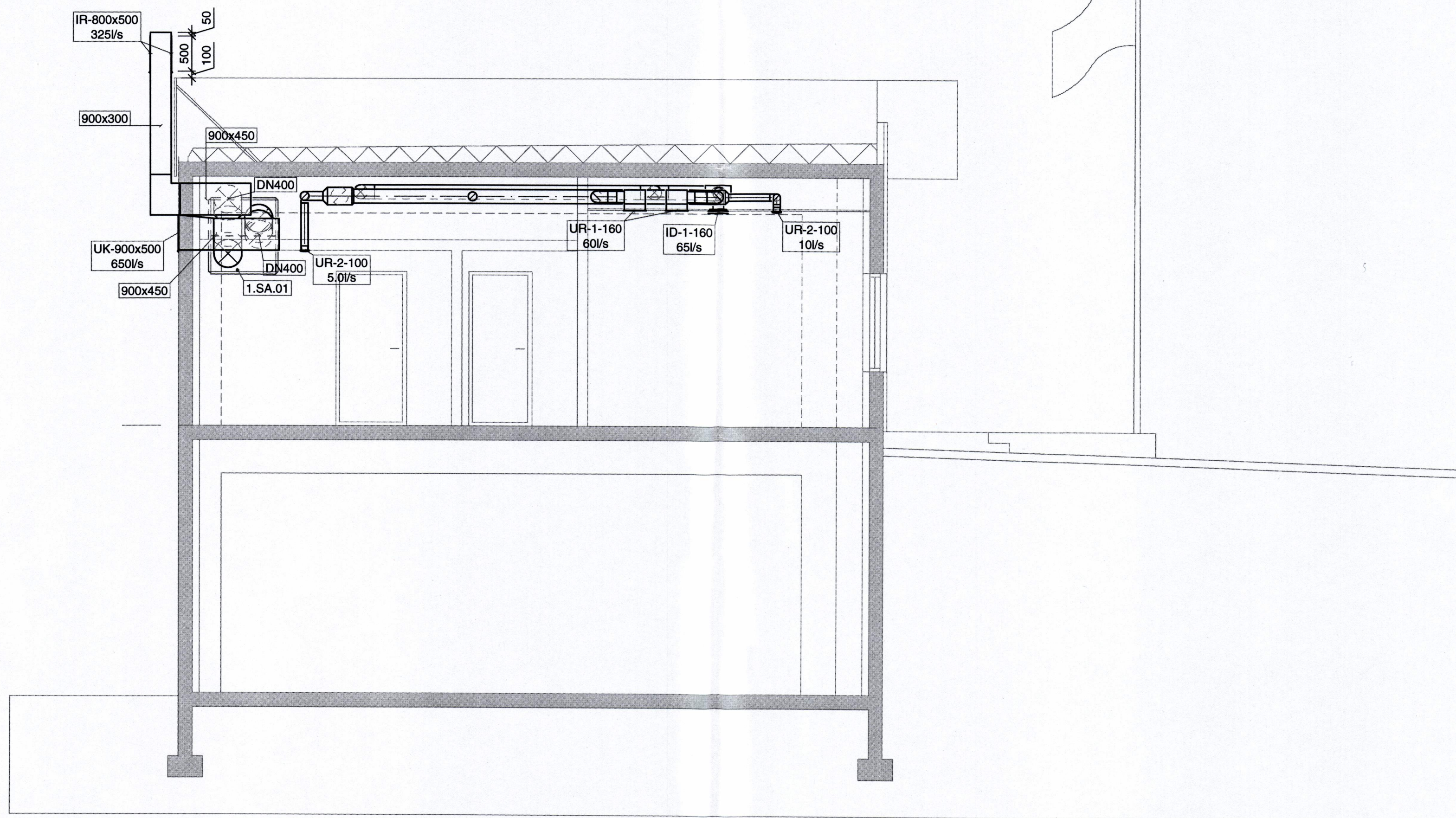
B SNIÐ L-501 1:50
