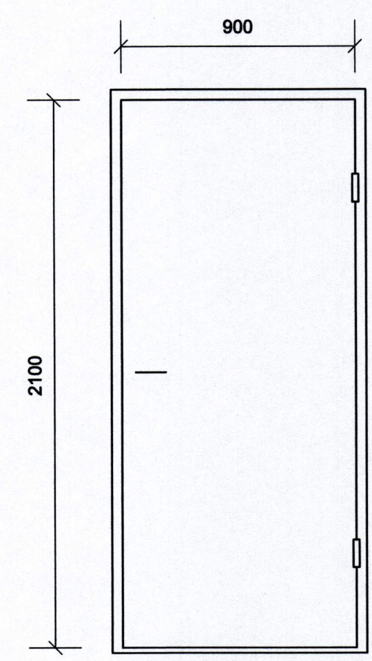
H-7, 2 stk.
