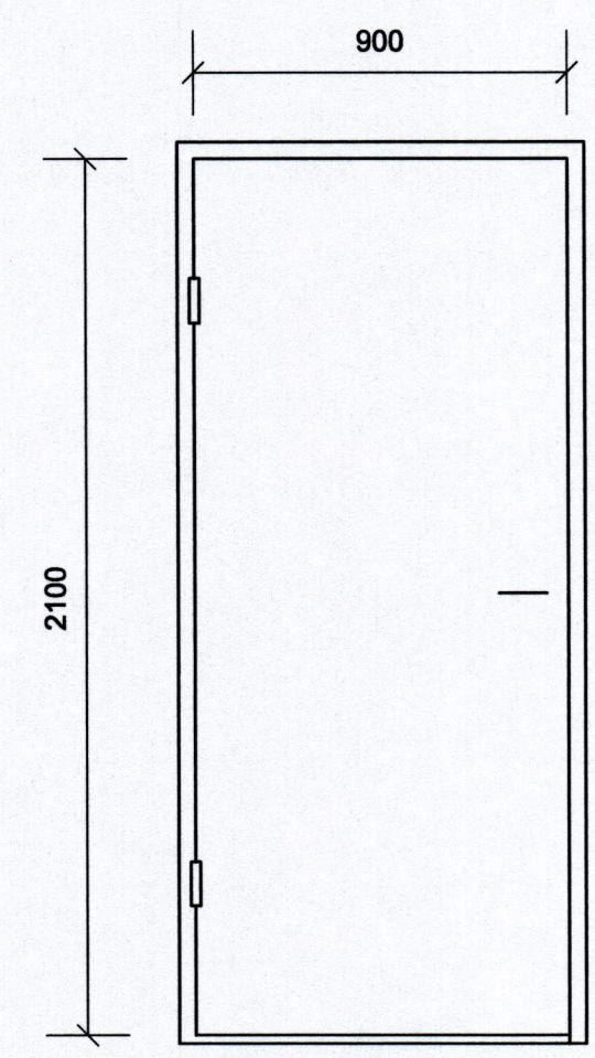
H-5, 2 stk.
