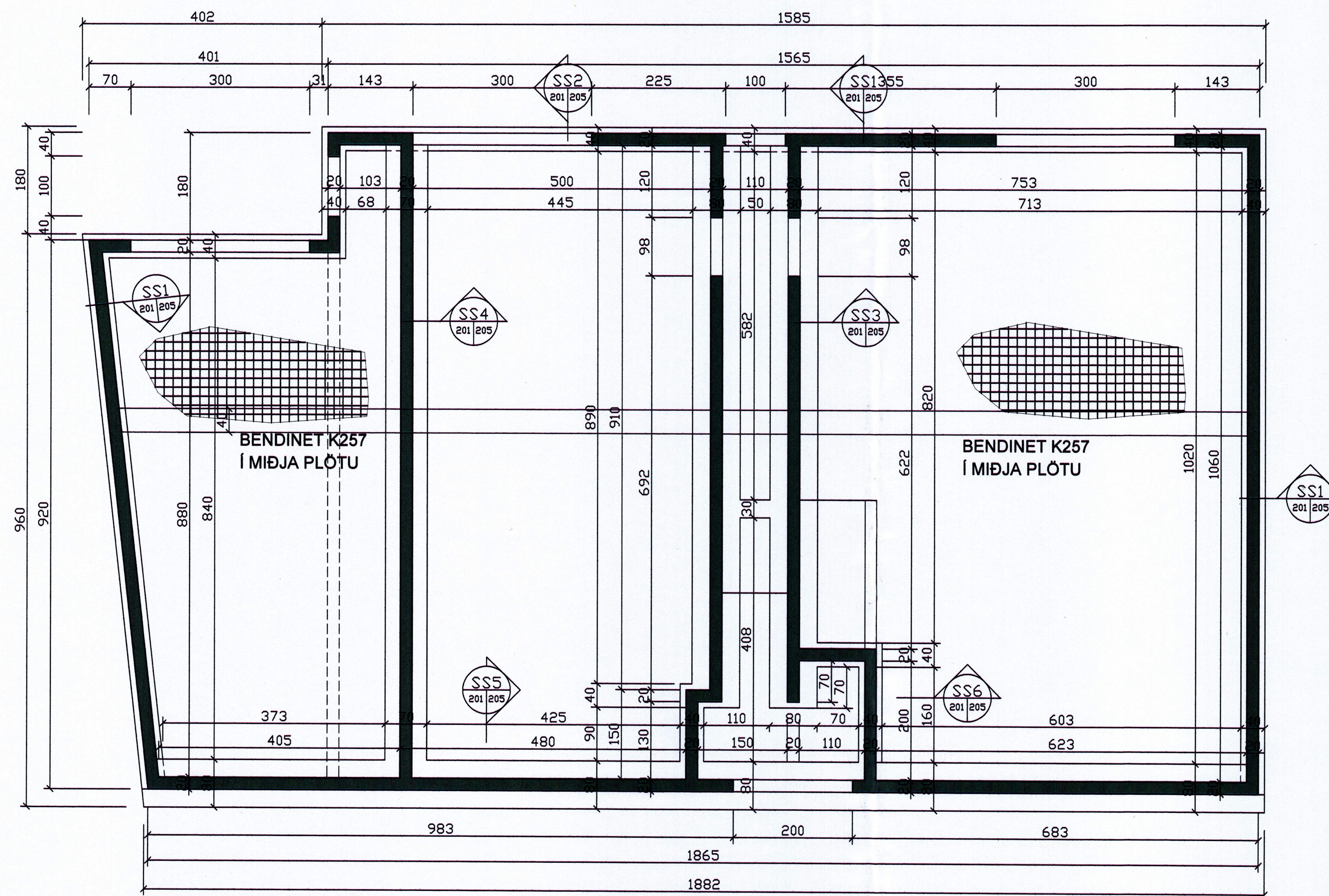
GRUNNMYND UNDIRSTÖÐUR
