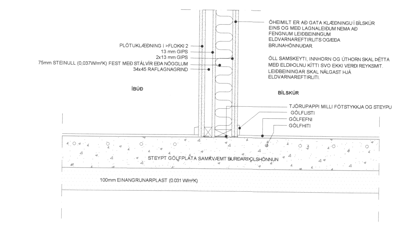
D3 SNIÐ - EI80 1:10
