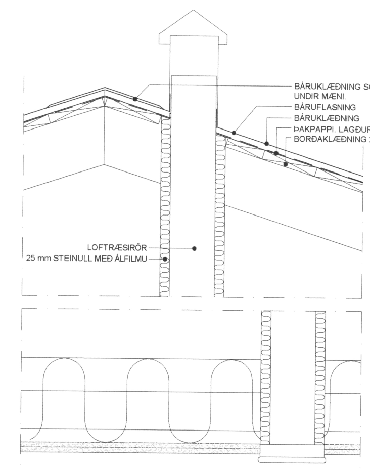
D5 DEILI - LOFTRÆSI RÖR Í GEGNUM ÞAK 1:10
