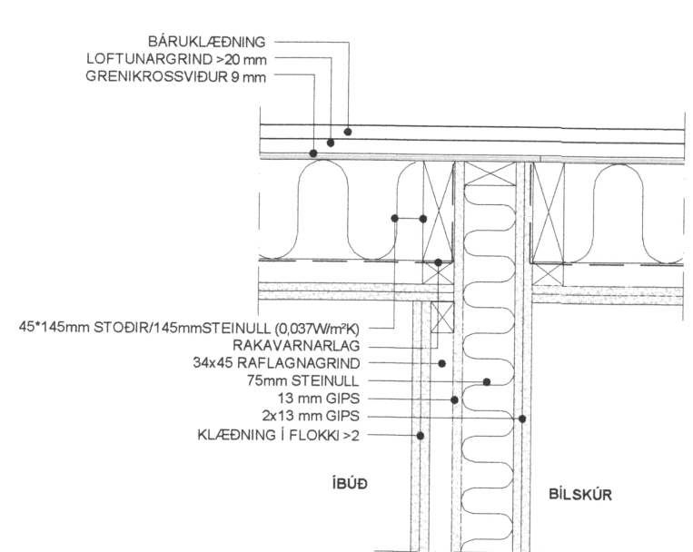
D4 DEILI - EI80 VEGGUR AD ÚTVEGG 1:10
