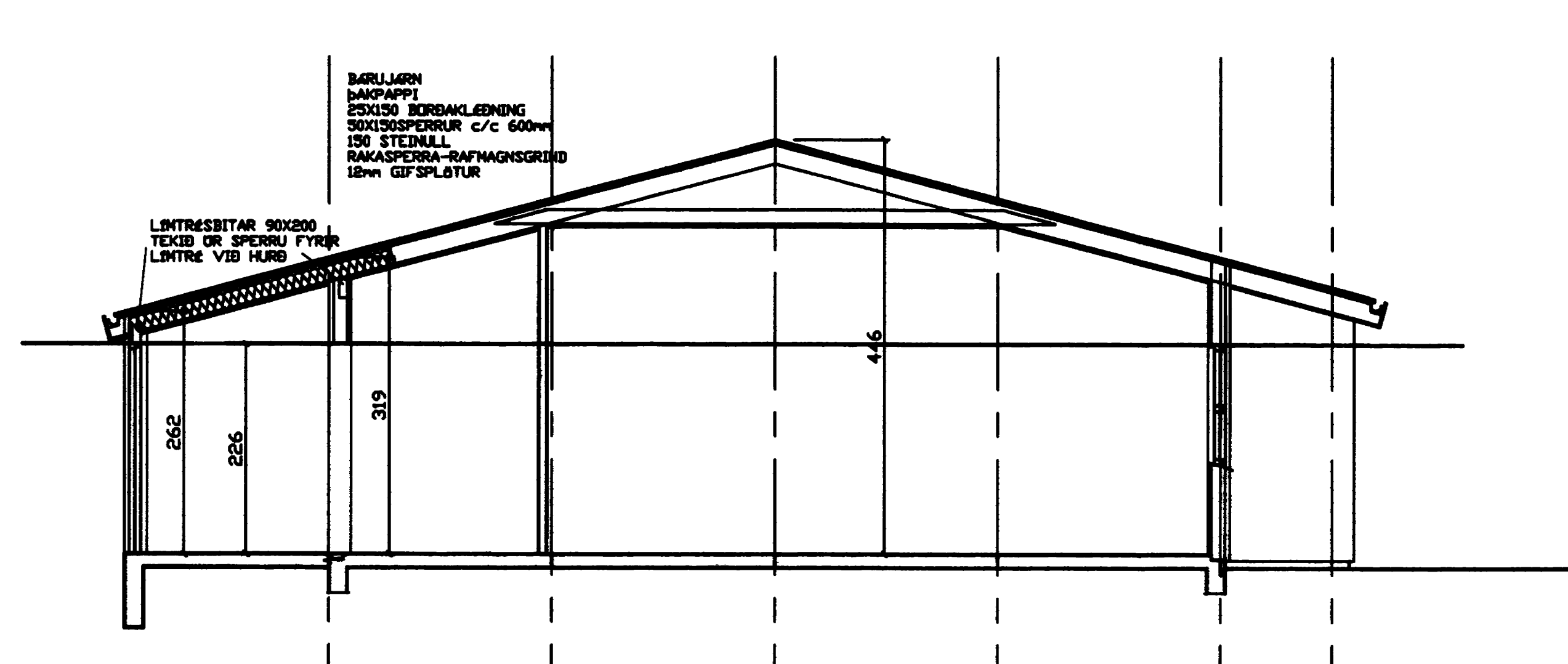
ÞVERSNIÐ M=1:100
