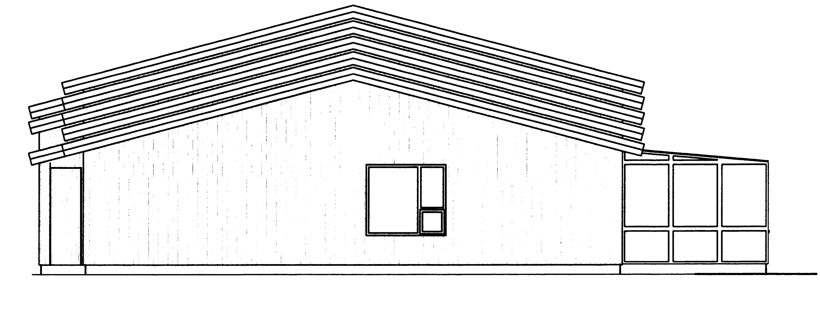
NORDERHLID M=1:100
