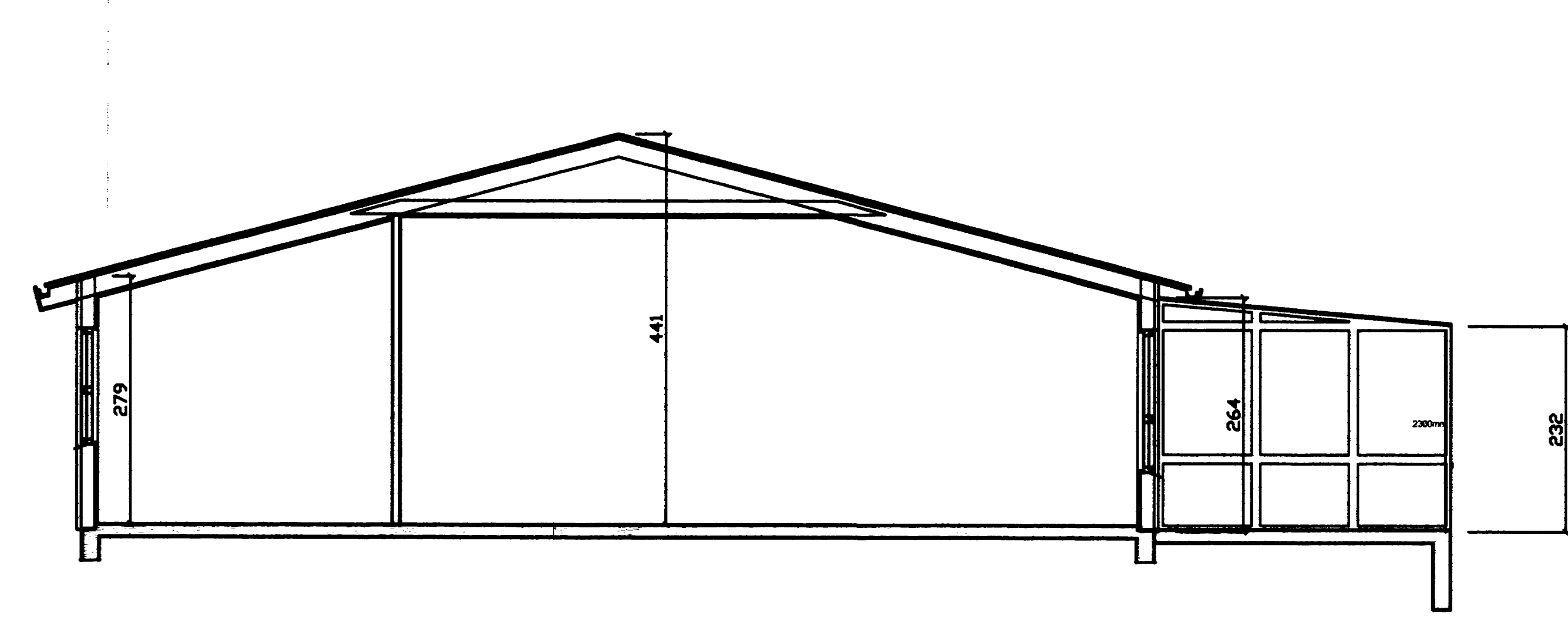
ÞVERSNIÐ M=1:100
