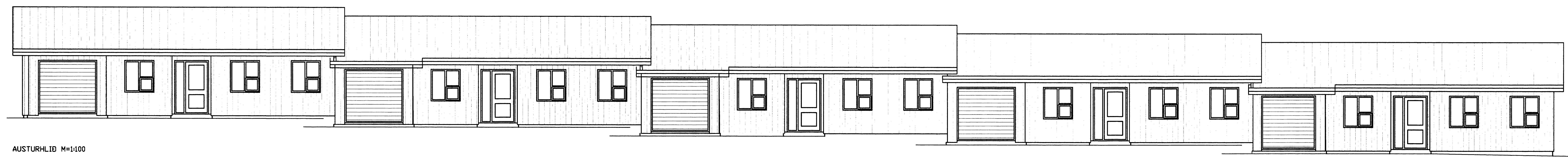
AUSTURHLID M=1:100
