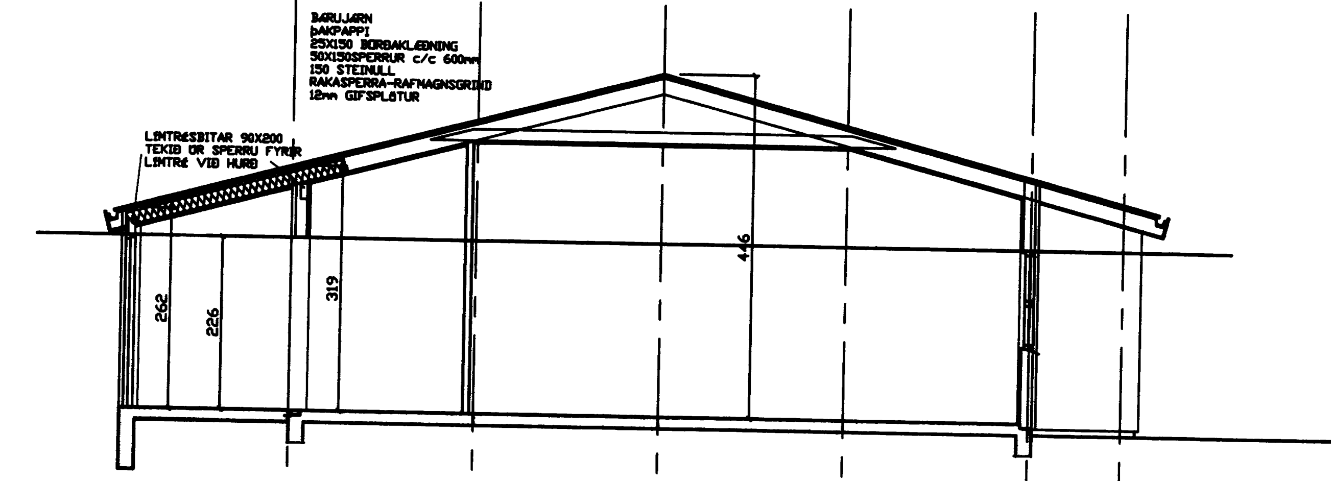
ÞVERSNIÐ M=1:100
