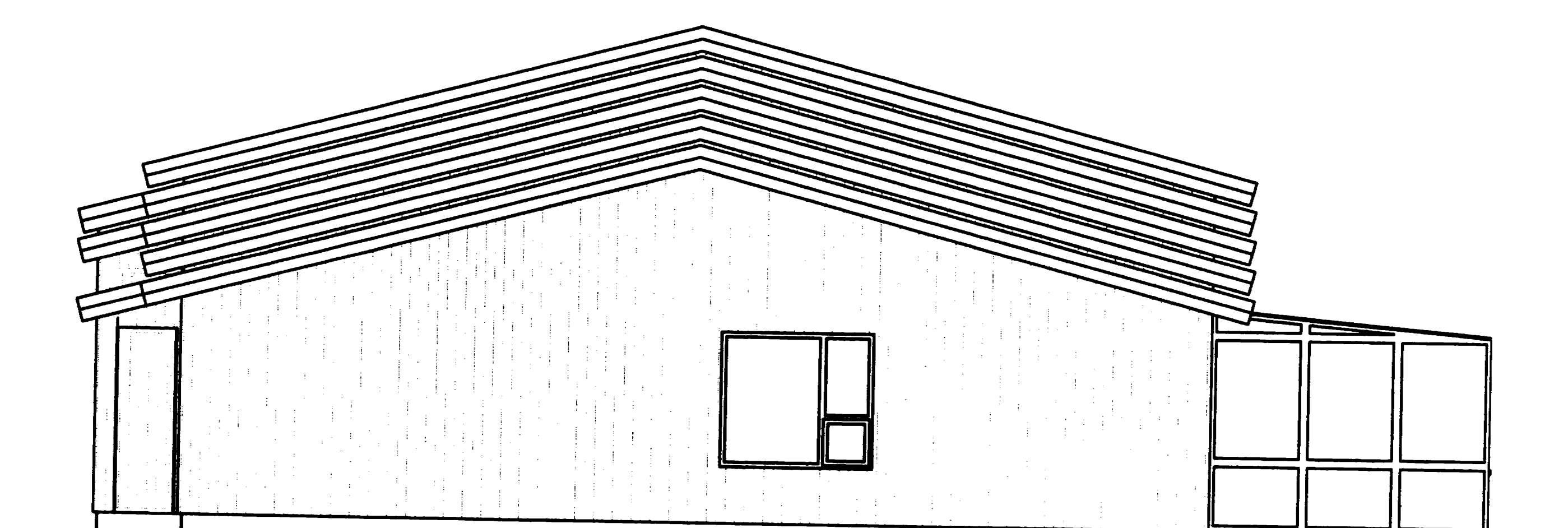
NORÐURHLID M=1:100
