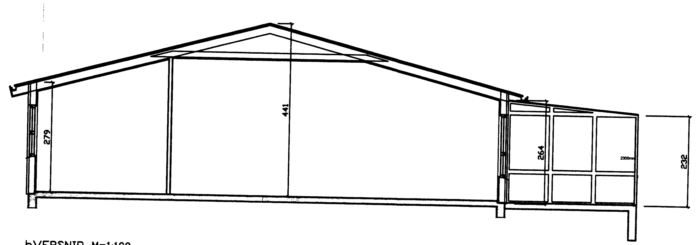
ÞVERSNIÐ M=1:100
