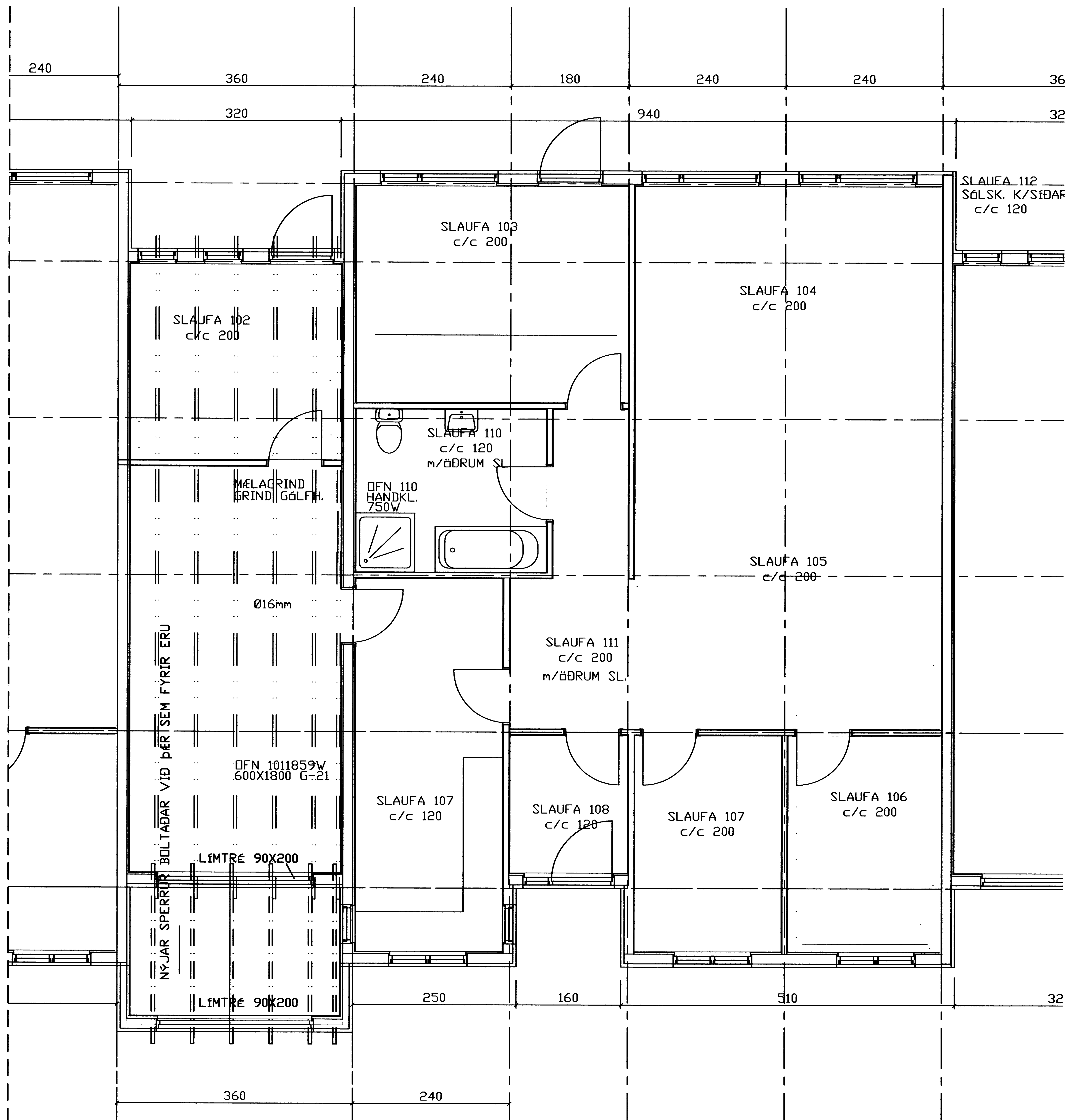
GRUNNMYND M=1:50
